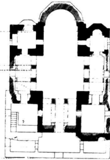
Κάτοψις Jerphanion. Εἰκ. 17. Ναὸς Ἁγ. Κλή- μεντος Ἀγκύρας. Κλ. 1:50
