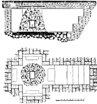
Εικ. 6. Κάτοψις και τομή του κάτωθεν της αγίας Τραπέζης του ναού του αγίου Δημητρίου Θεσσαλονίκης σταυρικού κτίσματος τού πιστευομένου ως τάφου του αγίου (κυρίως Μαρτύριου).
