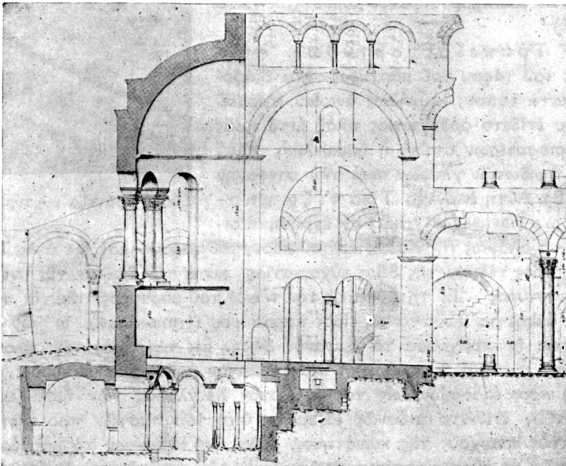
ΕΙΚ. 7. Τομή κατά μήκος του ιερού βήματος του ναού του αγίου Δημητρίου Θεσσαλονίκης, κάτωθεν του οποίου εκτείνεται ή Κρύπτη και τὸ Μαρτύριον του αγίου.
