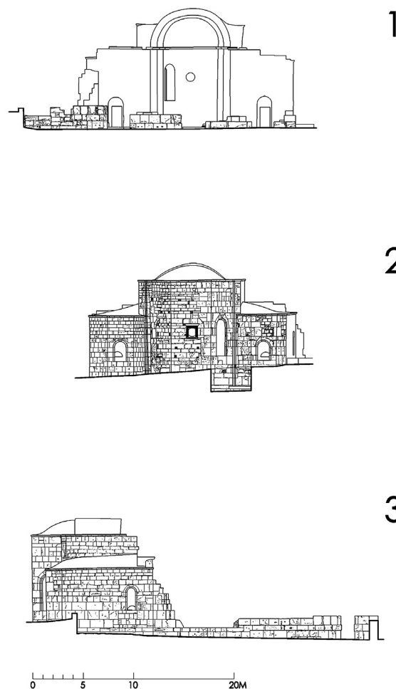
Εικ. 3. Γόρτυς, ναός Αγίου Τίτου. Αποτύπωση. Όψεις: 1. Δυτική όψη, 2. Ανατολική όψη, 3. Βόρεια όψη.
