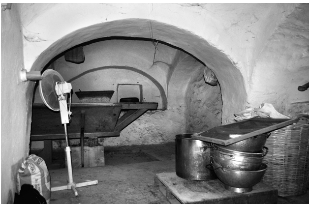
Εικ. 8. Μεγίστη Λαύρα, μαγκιπείο. Άποψη εσωτερικού κύριου χώρου προς βορειοανατολικά.
