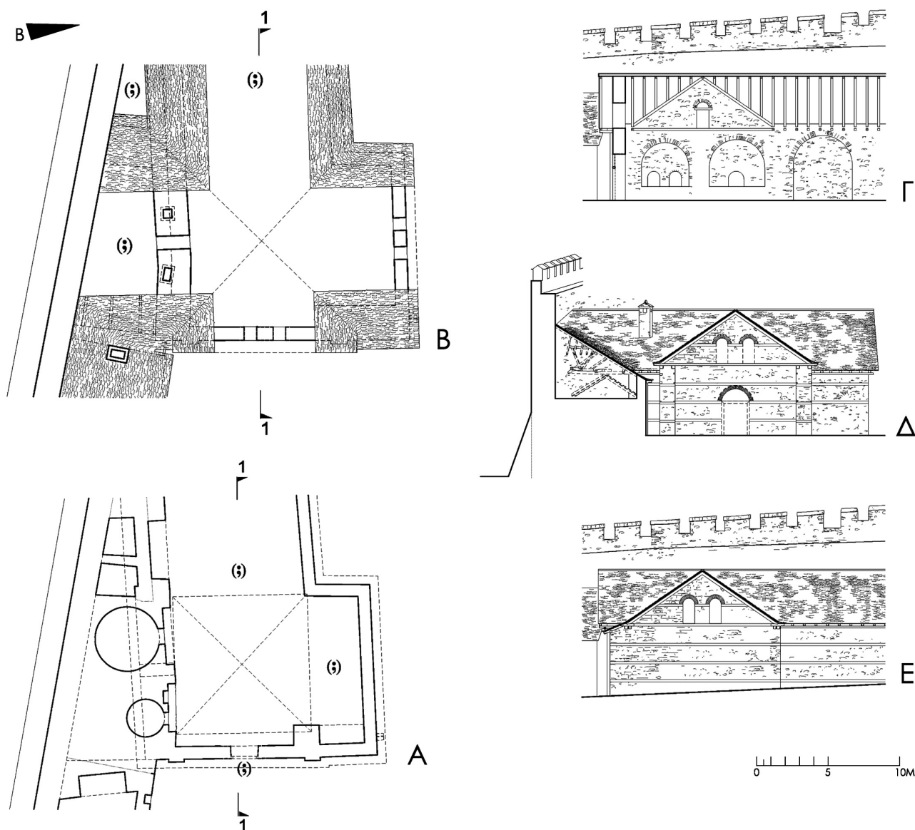
Εικ. 11. Μεγίστη Λαύρα, μαγκιπείο. Αναπαράσταση. Α. Κάτοψη 1, Β. Κάτοψη 2, Γ. Τομή 1-1, Δ. Ανατολική όψη, Ε. Βόρεια όψη.
