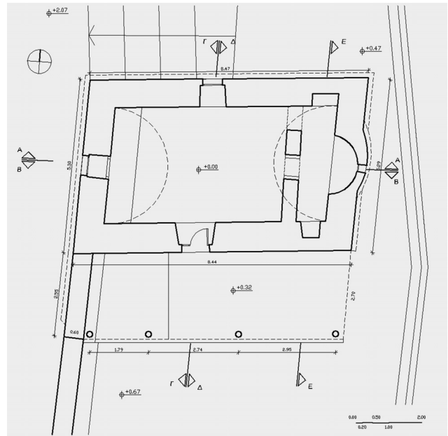
Εικ. 2. Ροεινό, ναός Παναγίας. Κάτοψη.
