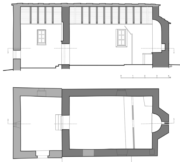
Εἰκ. 2. Κάτω Μερόπη, ναὸς Κοιμήσεως Θεοτόκου. Κάτοψη καὶ κατὰ μῆκος τομή.
