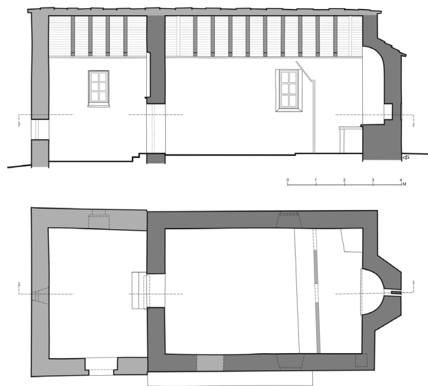
Εικ. 2. Κάτω Μερόπη, ναός Κοιμήσεως Θεοτόκου. Κάτοψη και κατά μήκος τομή.
