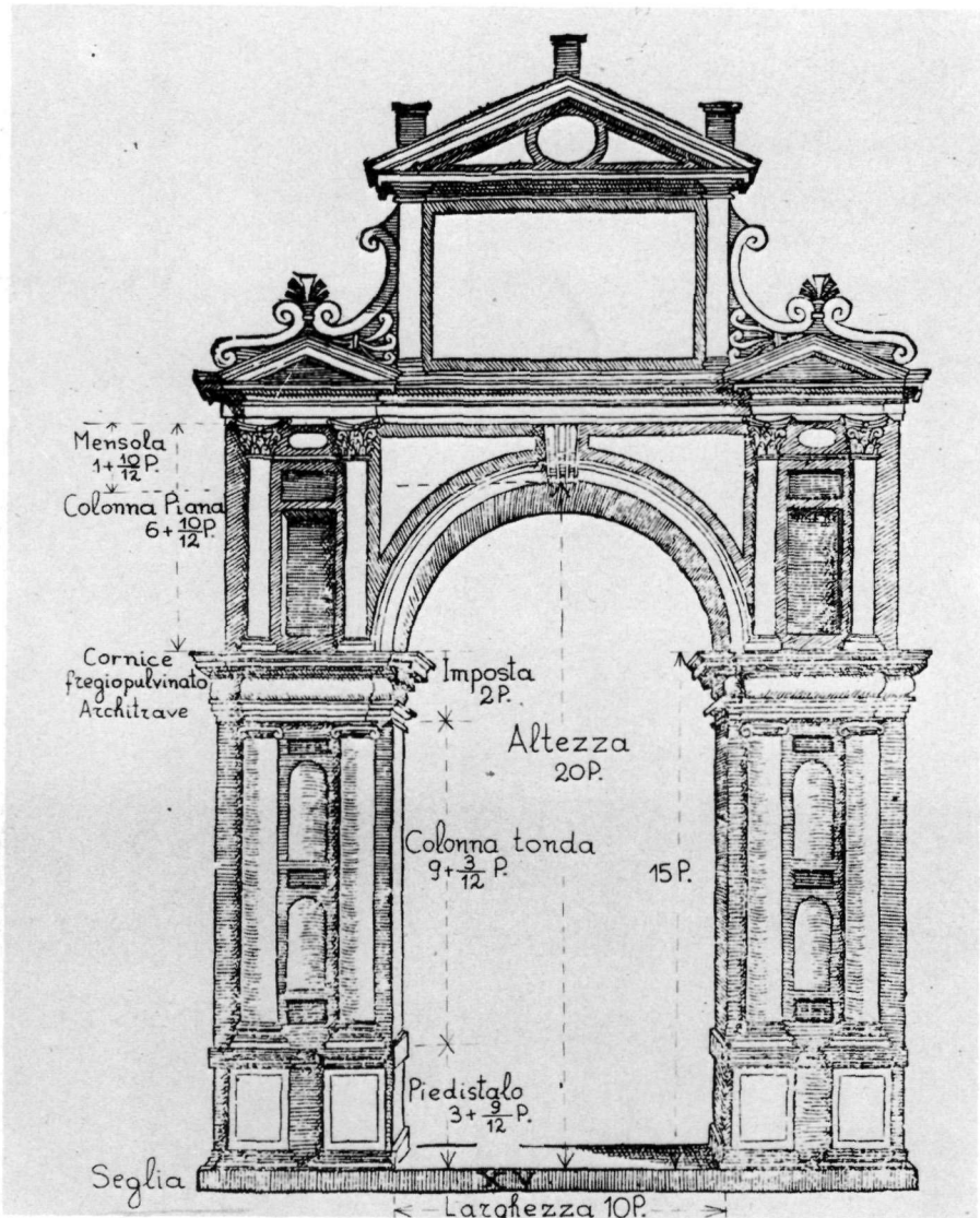
Sebastiano Serlio, «Libro straordinario». Porta XV. (Οί ένδείξεις τών διαστάσεων έχουν προστεθεί από τόν συγγραφέα, σύμφωνα με τó κείμενο τού Serlio).
