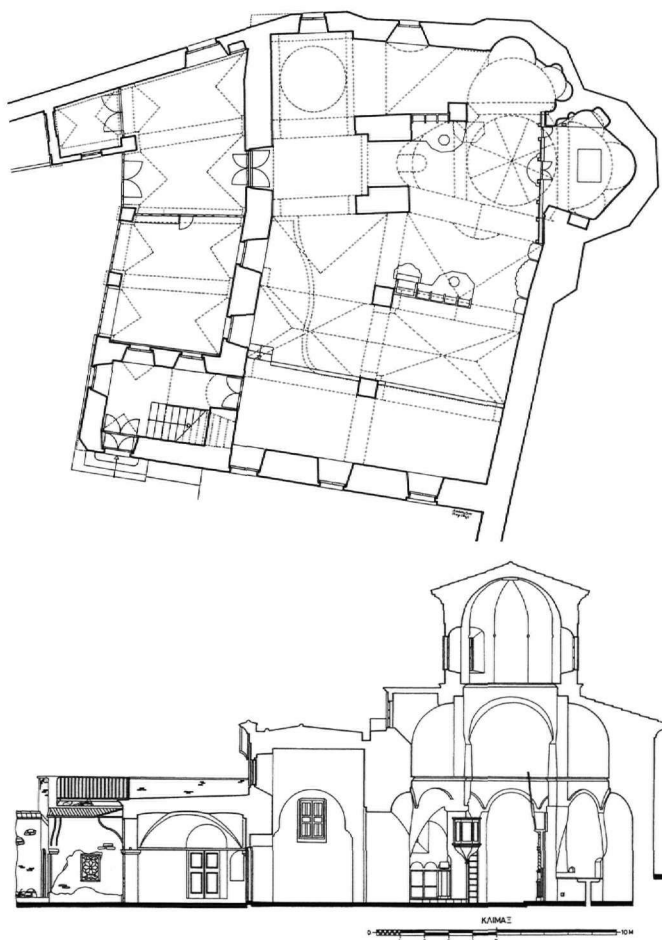
Εἰκ. 3. Παναγία τοῦ Μοναχλίου. Κάτοψη καὶ κατὰ μῆκος τομή. Ὑφισταμένη κατάσταση (σχέδ. Ἀ. Πορίδης).
