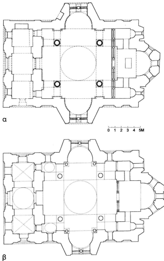
Εικ. 4. α. Καθολικό μονής Βατοπεδίου. Αναπαράσταση: Κάτοψη. β. Καθολικό μονής Ιθρών. Αναπαράσταση: Κάτοψη (βάσει σχεδίων Π. Μυλωνά).
