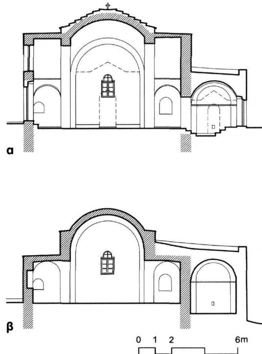
Εικ. 3. Κάλυμνος. Άγιοι Απόστολοι. Τομή κατά πλάτος προς Α. και στο ύψος του ανατολικού σταυρικού σκέλους.
