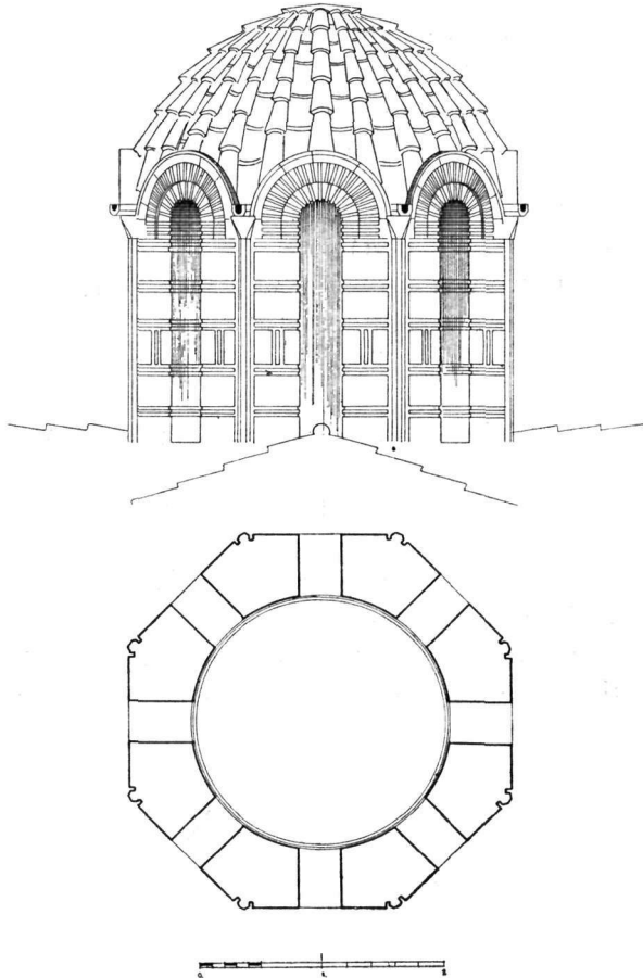
Εἰκ. 7. Ναὸς Ἁγ. Ἀσωμάτων. Τομὴ καὶ ὄψεις τοῦ τροῦλλου.
