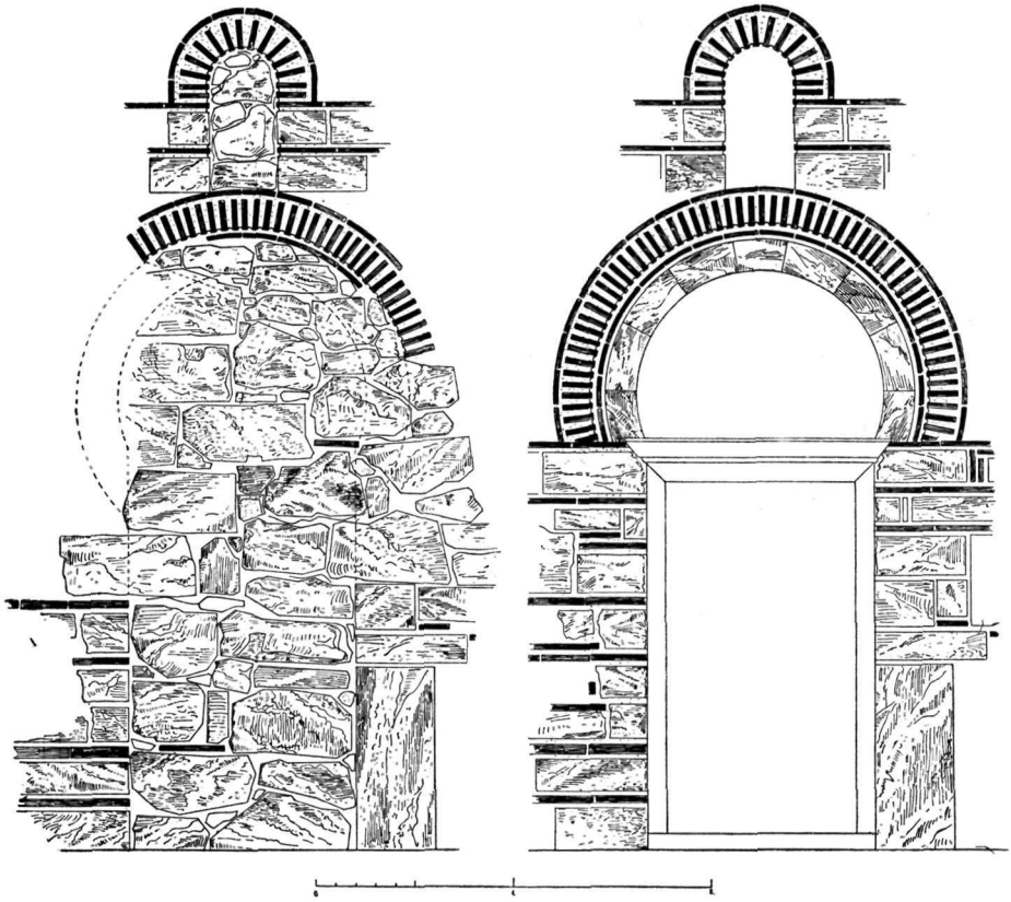
Εἰκ. 3. Θύρα μὲ πεταλόμορφον τόξον εἰς τὴν βορείαν πλευρὰν τοῦ νάρθηκος. Μορφή, τὴν ὁποίαν εἶχε κατὰ τὴν εὐρεσίαν της, καὶ ἀποκατάστασις τοῦ ἀρχικοῦ της σχήματος.
