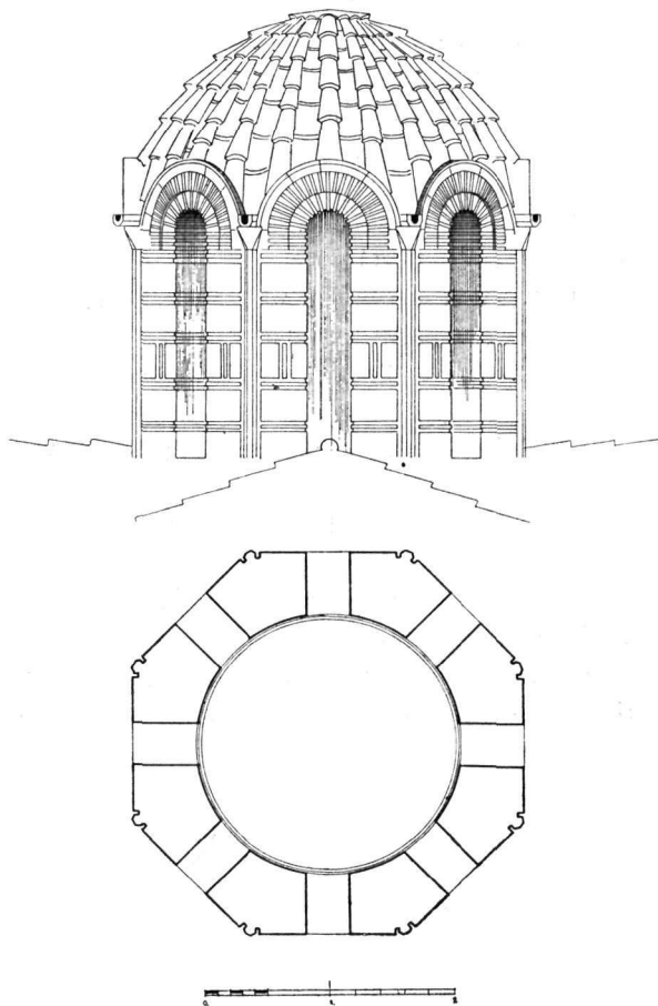
Εἰκ. 7. Ναὸς Ἀγ. Ἀσωμάτων. Τομὴ καὶ ὄψεις τοῦ τρούλλου.
