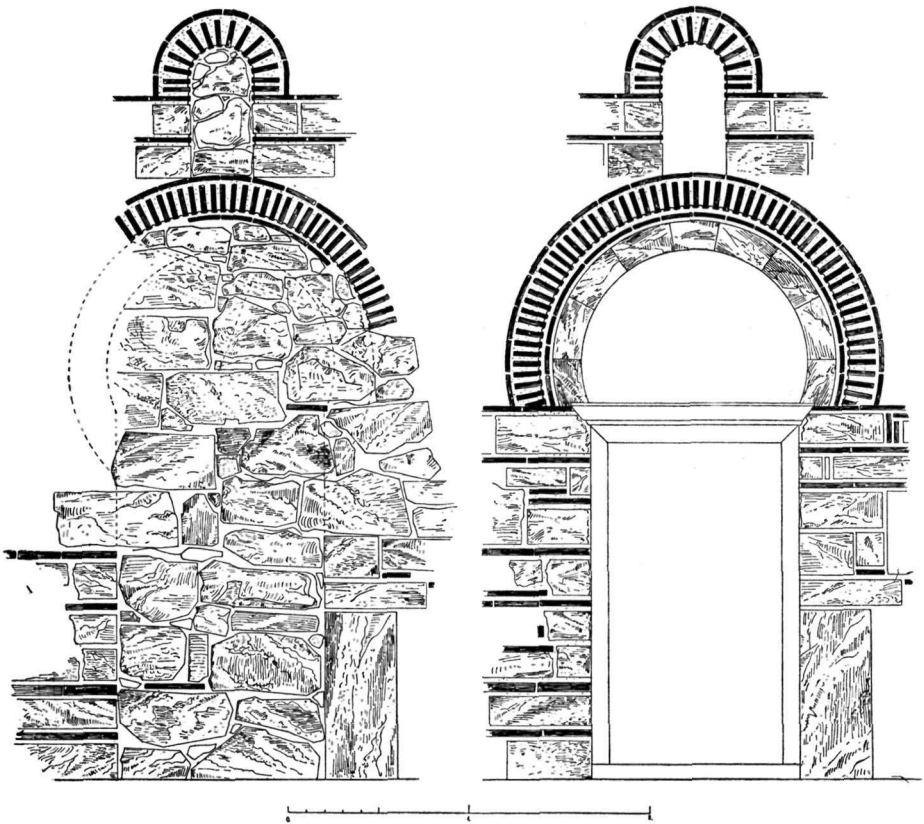
Εἰκ. 3. Θύρα με πεταλόμορφον τόξον εἰς τὴν βορείαν πλευρὰν τοῦ νάρθηκος. Μορφή, τὴν ὁποίαν εἶχε κατὰ τὴν εὕρεσίν της, καὶ ἀποκατάστασις τοῦ ἀρχικοῦ της σχήματος.
