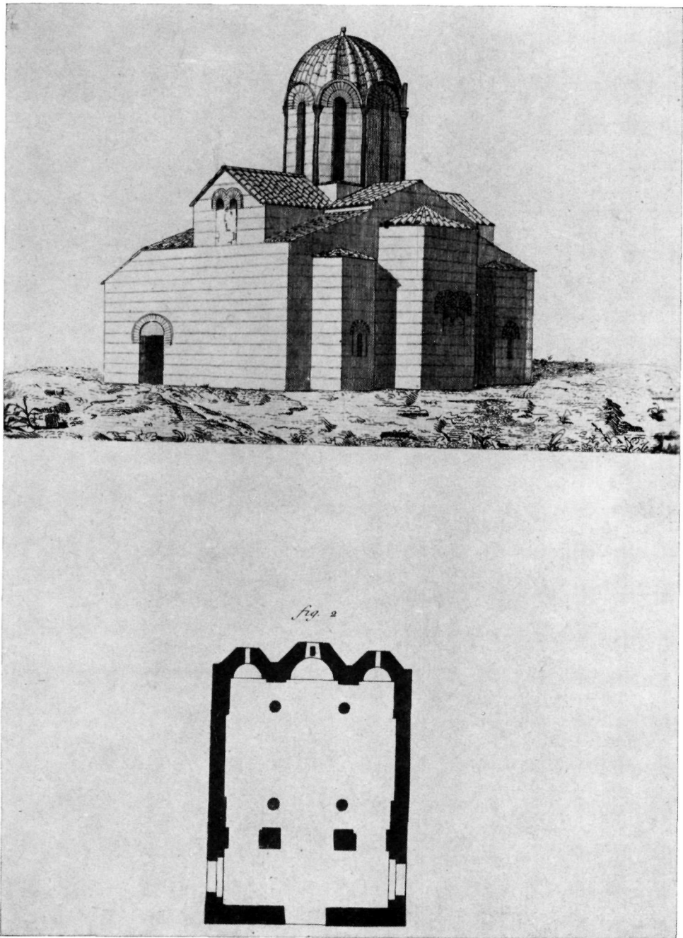
Κάτοψις καὶ ἀναπαράστασις τοῦ μνημείου ὑπὸ τοῦ Α. Couchaud (1842). ΝΑΟΣ ΑΓΙΩΝ ΑΣΩΜΑΤΩΝ
