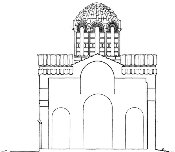
Εἰκ. 6. Τομή κατὰ πλάτος τοῦ κυρίως ναοῦ καὶ τοῦ νάρθηκος μετὰ τὴν ἀποκατάστασιν.
