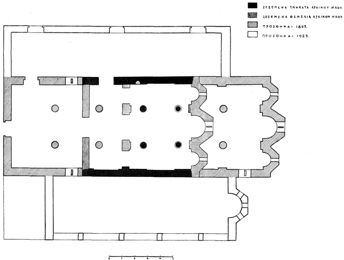
Είχ. 1. Ναός Ἀσωμάτων. Κάτοψις τοῦ μνημείου πρὸ τῶν ἐργασιῶν.
