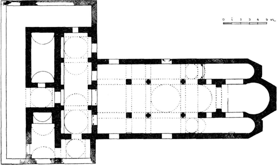
Εἰκ. 2. Κάτωψις τῆς Ἐπισκοπῆς Δαμαλᾶ κατὰ G. Welter.
