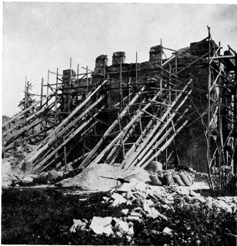
2. Ἰσχυρά ἱκρίσματα διὰ τὴν ἐπαναφορὰν τοῦ δυτικοῦ τοίχου εἰς τὴν κατακόρυφον.
