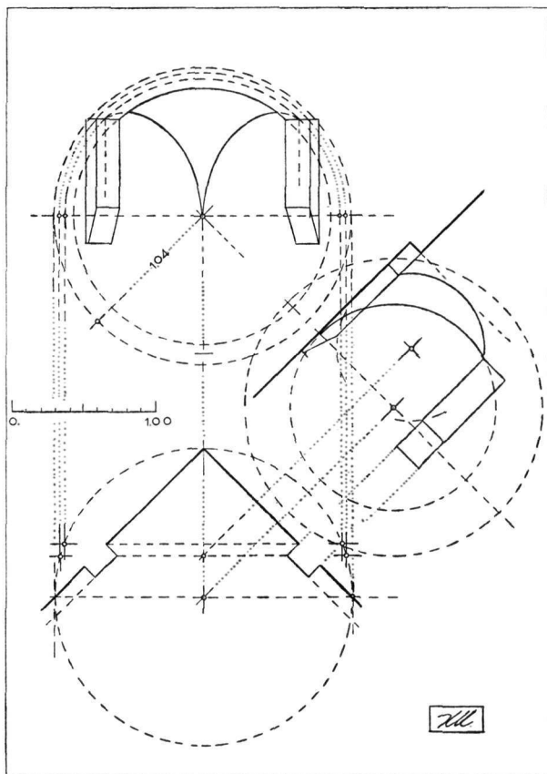
Εἰκ. 11. Ἁγίος Ἰωάννης Κέρους. Γεωμετρικὴ ἐρμηνεῖα τῆς κατασκευῆς τῶν ἡμιχωνίων. Κάτοψις, ὄψις πλαγία καὶ ὄψις κατὰ τὴν διαγώνιον.
