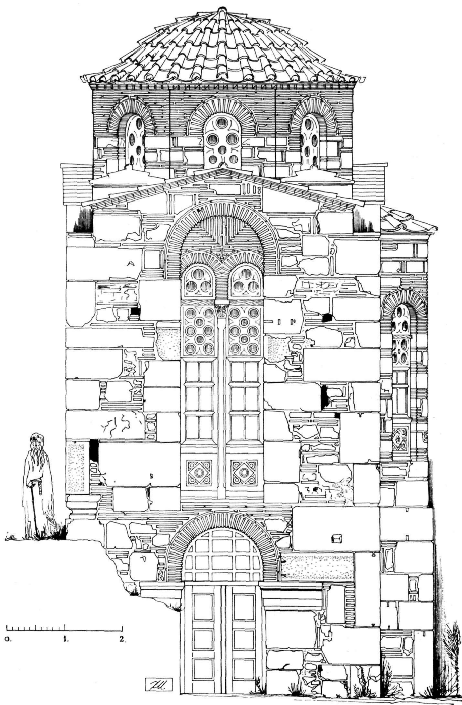
Εἰκ. 5. Ναῖσκος Ὁσίου Λουκά. Ἀναπαράστασις τῆς ἀρχικῆς μορφῆς τοῦ μνημείου. Νοτία ὄψις.
