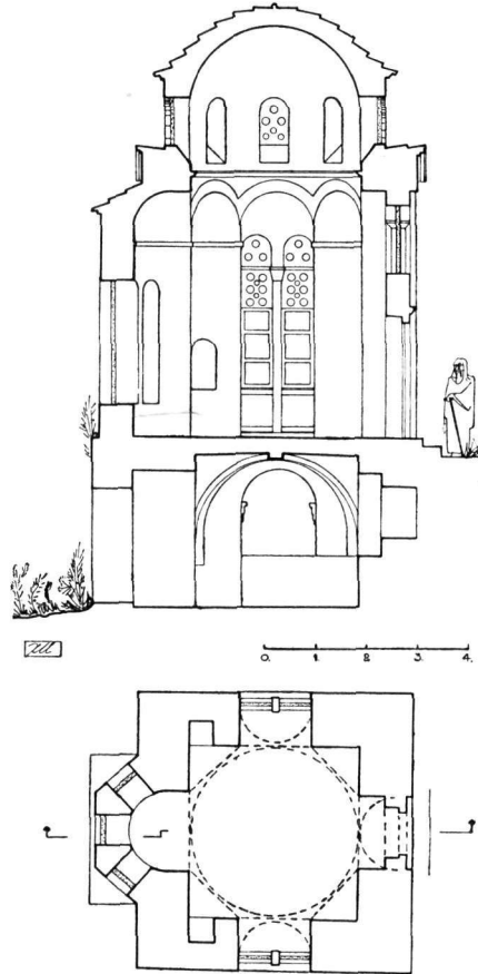
Εἰκ. 4. Ναῖσκος Ὁσίου Λουκά. Ἀναπαράστασις τῆς ἀρχικῆς μορφῆς τοῦ μνημείου. Κάτοψις τοῦ ὁρόφου καὶ τομὴ κατὰ μήκος.
