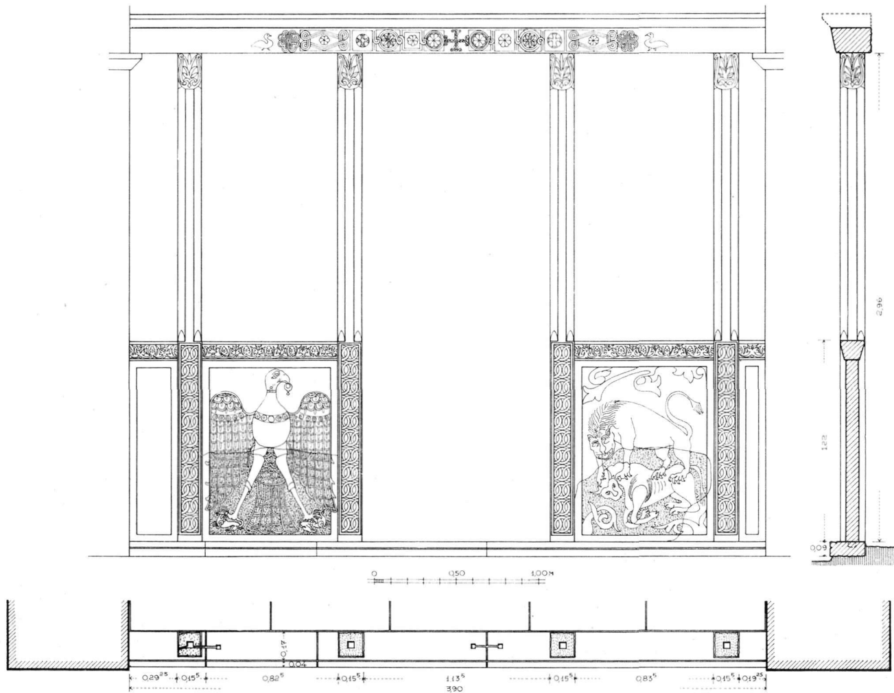
Εικ. 1. Κάτοπις τοῦ στυλοβάτου καὶ ἀναπαράστασις τῆς ὀρθώσεως τοῦ μέσου τμήματος τοῦ τέμπλου τῆς Ἁγ. Θεοδώρας Ἄρτιας. Εἰς τὸ δεξιὸν πλάγιον, κατακόρυφος τομὴ τοῦ τέμπλου.
