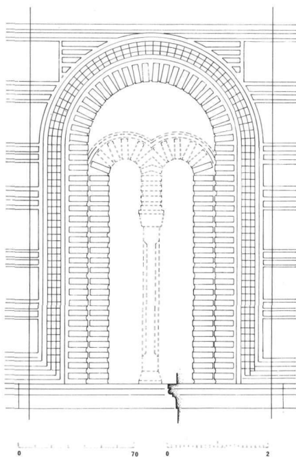
Εἰκ. 13. Θεοτόκος Ἀηλίου. Τό δίλοβο παράθυρο τῆς κεντρικῆς κόγχης τοῦ ἱεροῦ, σέ ἀναπαράσταση.
