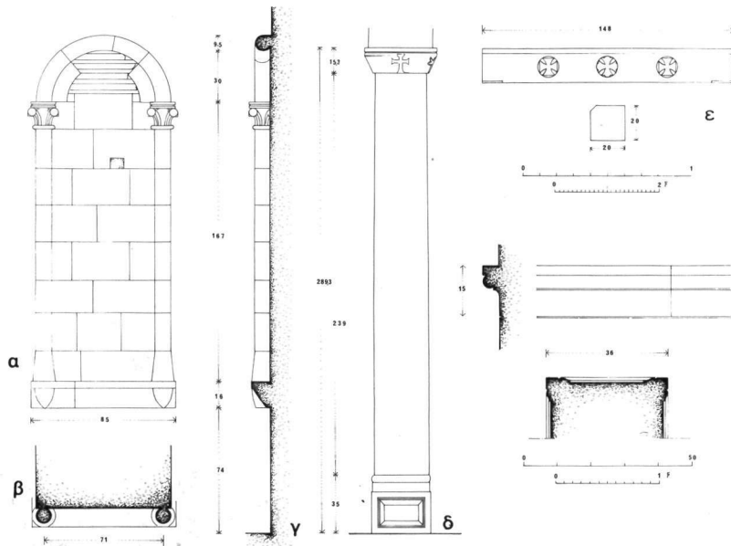
Είκ. 4. Θεοτόκος Ἀνηλίου. Λεπτομέρειες σέ ἀναπαράσταση: α. Προσκυνητᾶρι πεσσοῦ τοῦ ἱεροῦ σέ κάτοψη καί τομή. β. Ἐνας ἀπὸ τοὺς κίονες. γ. Τὸ ὑπέρθυρο σέ ὄψη καί τομή. δ. Ὁ πῶρινος κοσμητὴς τοῦ ἱεροῦ σέ ὄψη καί τομή. ε. Τὸ δάθρο τοῦ κίονος σέ τομή.
