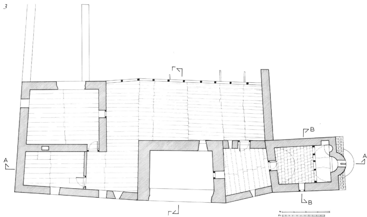
Εικ. 2-3. Μονή Τορνικίου. Κάτοψη ισογείου και ορόφου.
