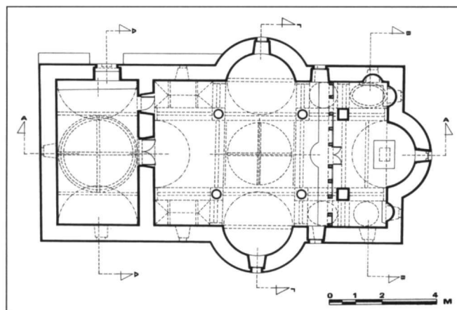
Είκ. 2. Άγιος Ιωάννης ο Θεολόγος Ζάρκων. Κάτοψη.
