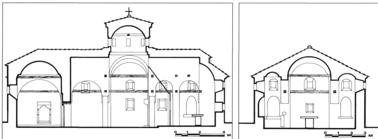
Εἰκ. 3-4. Ἁγιος Ἰωάννης ὁ Θεολόγος Ζάκρου. Τομή κατά μήκος καὶ ἐγκάρσια τομή στό ἱερό βῆμα, ἀντίστοιχα.
