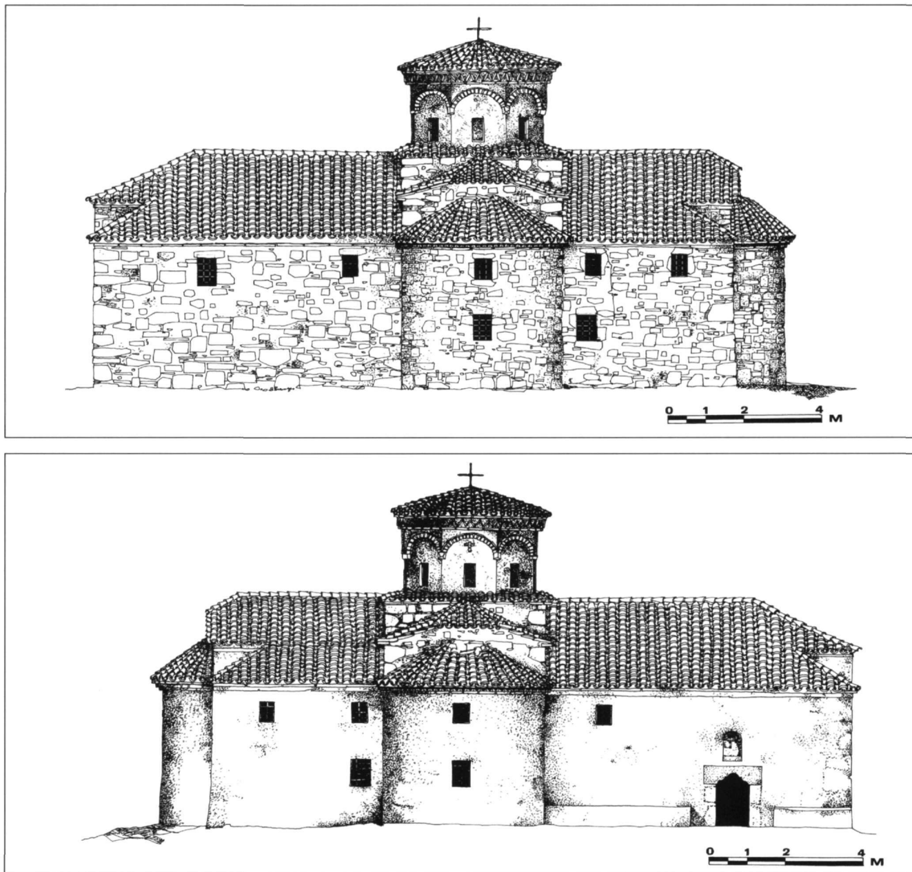
Εικ. 10-11. Ἅγιος Ἰωάννης ὁ Θεολόγος Ζάκχον. Νότια καί βόρεια ὄψη, ἀντίστοιχα.
