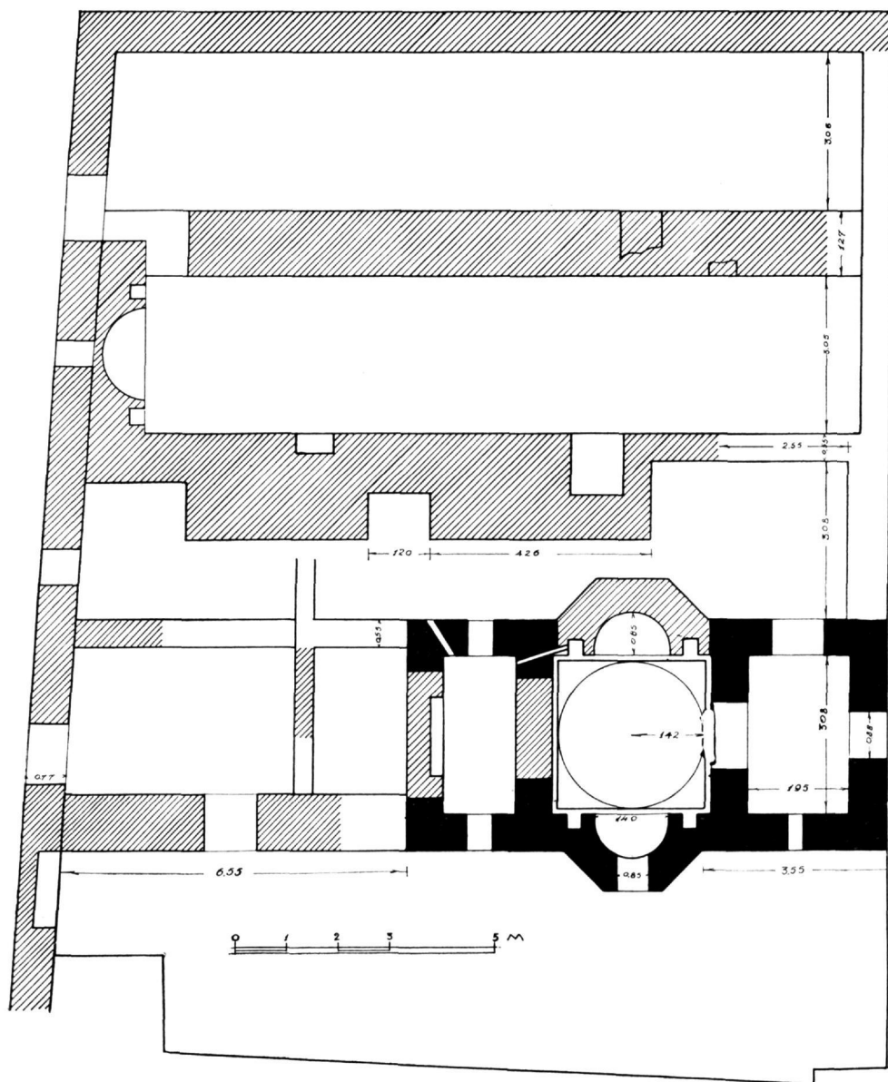
Εἰκὼν 1.— Κάτοψις τοῦ νοτιανατολικοῦ διαμερίσματος τῆς Μονῆς Καισαριανῆς, ἔνθα περικλείεται νῦν τὸ ἅγιασμα.
