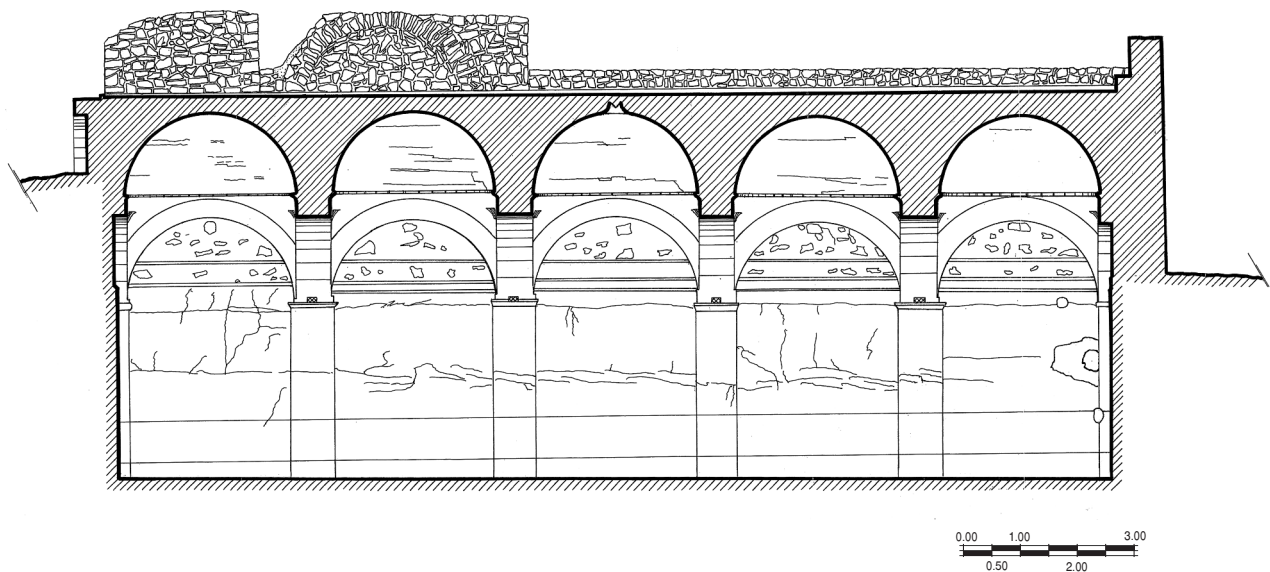
Εικ. 4. Όψη και τομή κατά μήκος της κινστήρας.
