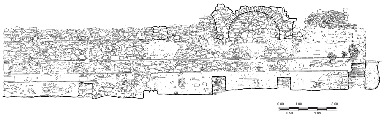
Εικ. 6. Η βόρεια όψη της κινστέρνας.
