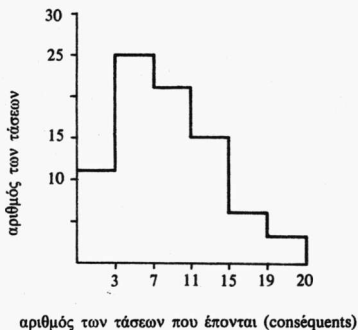
Γραφική παράσταση 4: Ιστόγραμμα των τάσεων που έπονται (conséquents)
