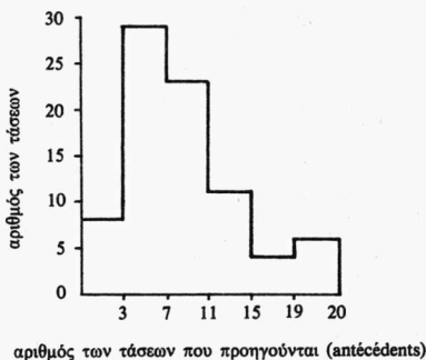
Γραφική παράσταση 3: Ιστόγραμμα των τάσεων που προηγούνται (antécédents)
