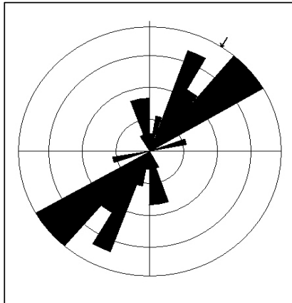
Σχήμα 13. Ροδοδιάγραμμα κατευθύνσεων των ρεμάτων ριπιδίου Καλής Βρύσης.
