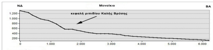
Σχήμα 9. Μορφολογική τομή κατά μήκος του ριπιδίου της Καλής Βρύσης.
