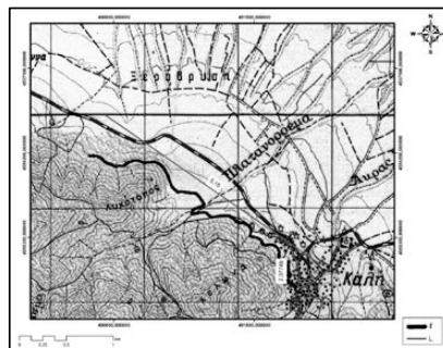
Σχήμα 2. Εφαρμογή του δείκτη smf στους πρόποδες του Μεινοϊκίου όρους (στα πλαίσια αναγράφονται τα μήκη των l και L σε km)
