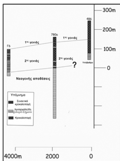
Σχήμα 5. Στρωματογραφική τομή στο ριπιδίο της Προσοτσάνης.
