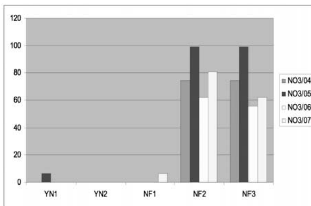
Fig. 7: NO 3 histogram.
