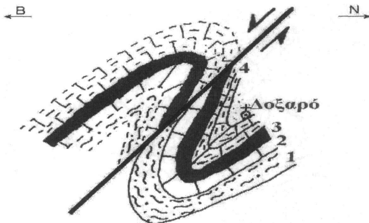
Σχήμα 2. Σχηματική απεικόνιση της γεωλογικής δομής και της αναστροφής των στρωμάτων στα Τάλαια όρη.
