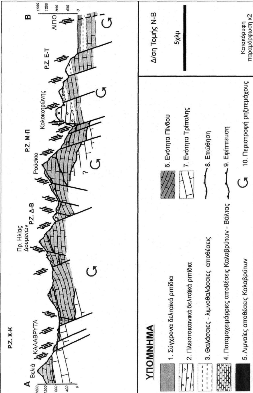
Εικ.2 .Απλοποιημένη γεωλογική τομή στο φύλλο ΑΙΓΙΟ, σε διεύθυνση Ν – Β.
