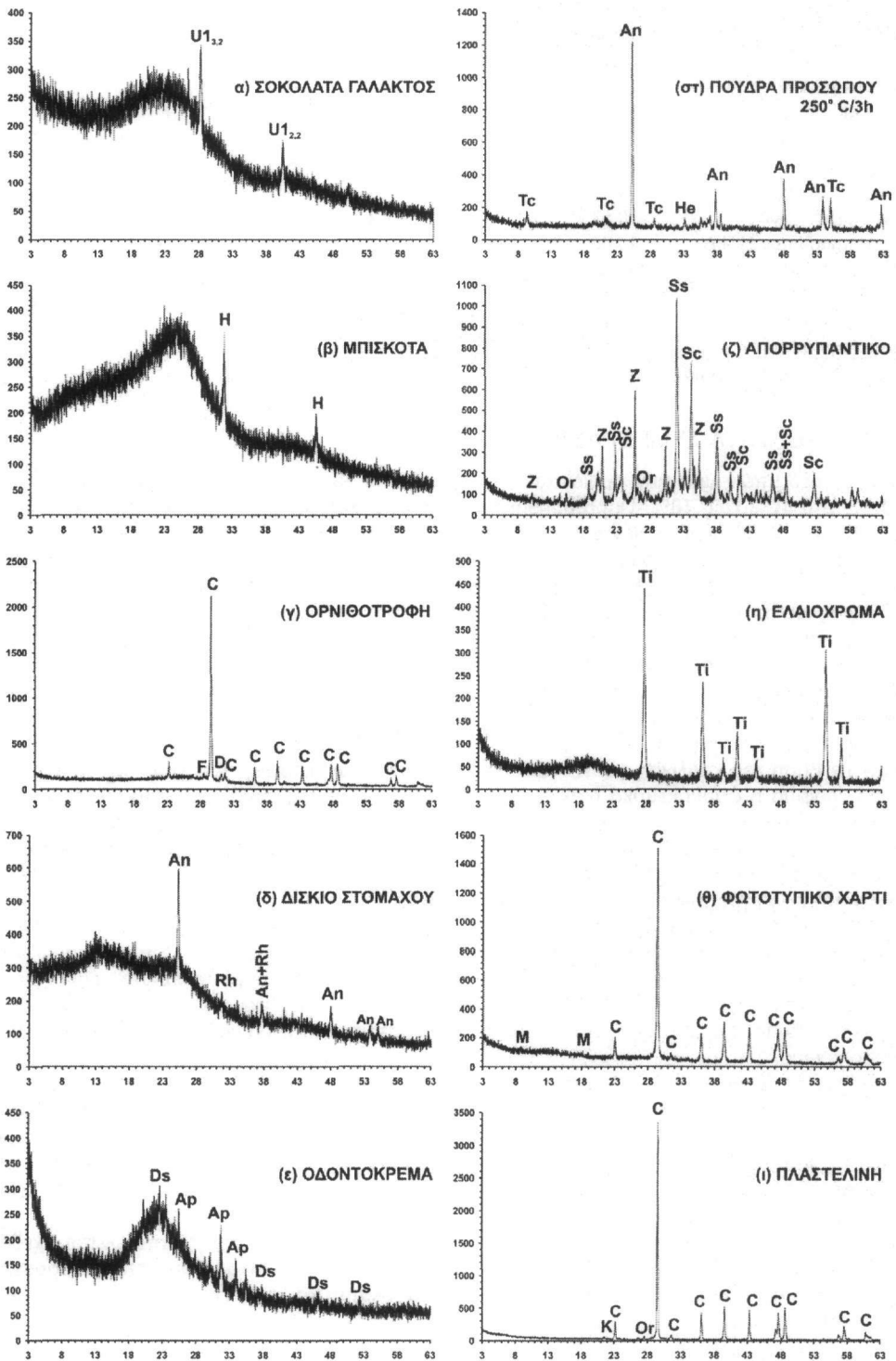
Σχήμα 1. Περιθλασιογράμματα στερεού υπολείμματος προϊόντων μετά από θέρμανση σε 350° C/3 h. Σύμβολα όπως στον Πίνακα 2.
