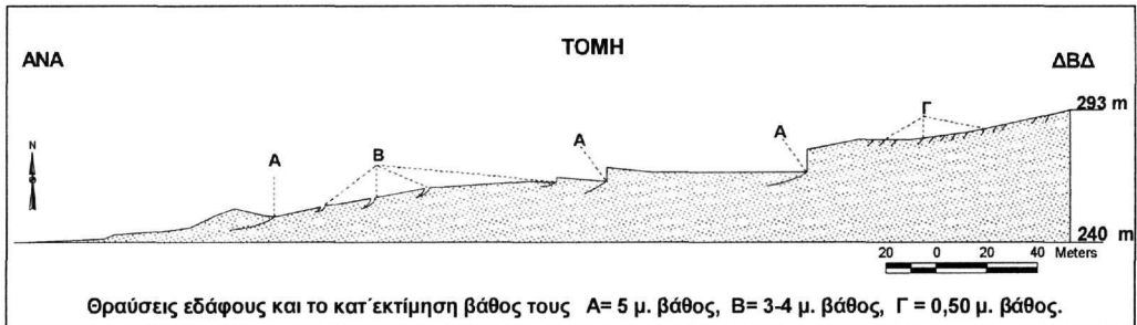
Σχήμα 4. Μορφολογική τομή κατά μήκος και περίπου στη διεύθυνση της κίνησης. Οι μεγαλύτερες αναβαθμίδες εκτιμάται ότι σχηματίστηκαν με παλαιότερες θραύσεις και αργές μετακινήσεις του εδάφους.
