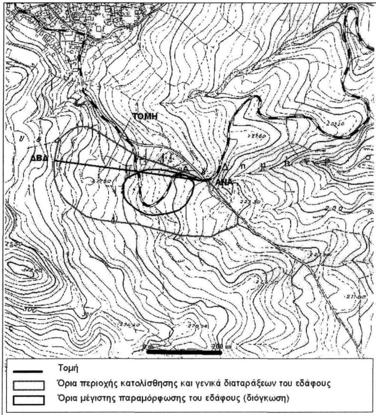
Σχήμα 3. Χάρτης περιοχής κατολίσθησης.
