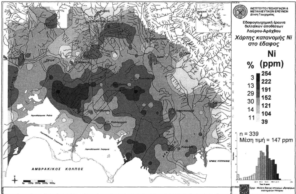
Σχήμα 2. Γεωχημικός χάρτης κατανομής Ni στο έδαφος.
