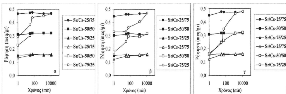
Σχήμα 7. Ρόφηση \text{Cs}^+ (μαύρα σύμβολα) και \text{Sr}^{2+} (κενά σύμβολα) α) σε φυσικό κλινοπτιλόλιθο β) σε κλινοπτιλόλιθο επεξεργασμένο με ακτινοβολία ηλεκτρονίων ( 10^{14} \text{ e/cm}^2 ) γ) σε κλινοπτιλόλιθο επεξεργασμένο με ακτινοβολία-γ (70Mrad). Τα ίδια σχήματα αναφέρονται σε διαλύματα αντίστοιχων αναλογιών για παράδειγμα ο μαύρος κύκλος αναφέρεται σε διάλυμα αναλογίας \text{Cs}^+/\text{Sr}^{2+}=75/25 και ο κενός κύκλος σε διαλύματα \text{Sr}^{2+}/\text{Cs}^+=75/25 . Συγκέντρωση διαλύματος 0,5xCEC.
