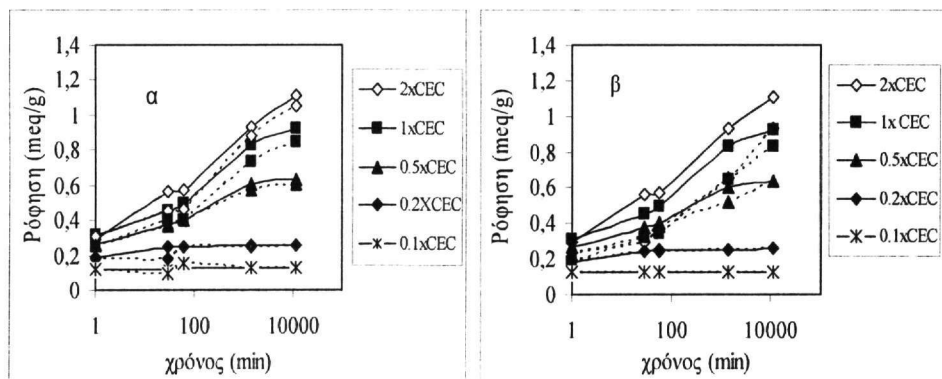
Σχήμα 3. Ρόφηση \text{Sr}^{2+} σε φυσικό κλινοπτιλόλιθο (συνεχής γραμμή) και α) σε κλινοπτιλόλιθο επεξεργασμένο με ακτινοβολία ηλεκτρονίων ( 10^{15} \text{ e/cm}^2 ) (διακεκομένη γραμμή) β) σε κλινοπτιλόλιθο επεξεργασμένο με ακτινοβολία γ (70Mrad) (διακεκομένη γραμμή) (άξονας x: χρόνος αντίδρασης, άξονας y: γραμμοισοδύναμα τα οποία ροφήθηκαν, για όλες τις συγκεντρώσεις έγινε αναγωγή ανά γραμμάριο κλινοπτιλόλιθου)
