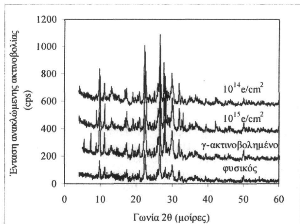
Σχήμα 1. Ακτινοδιαγράμματα φυσικού ζεολίθου, επεξεργασμένων με ακτινοβολία β ( 10^{14} \text{ e/cm}^2 έως 10^{15} \text{ e/cm}^2 ) και επεξεργασμένου με ακτινοβολία γ (70 Mrad) (άξονας x: ένταση ανακλώμενης ενέργειας σε κάθε πλεγματοειδές επίπεδο, άξονας ψ: γωνία αναλυτή κρυστάλλου.)
