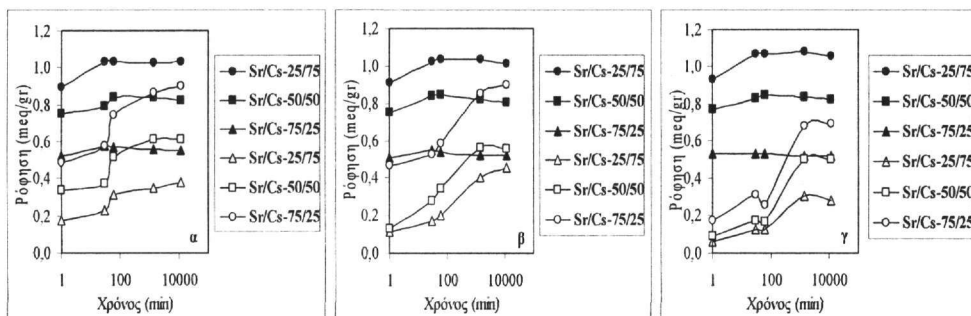
Σχήμα 6. Ρόφηση \text{Cs}^+ (μαύρα σύμβολα) και \text{Sr}^{2+} (κενά σύμβολα) α) σε φυσικό κλινοπτιλόλιθο β) σε κλινοπτιλόλιθο επεξεργασμένο με ακτινοβολία ηλεκτρονίων ( 10^{14} \text{ e/cm}^2 ) γ) σε κλινοπτιλόλιθο επεξεργασμένο με ακτινοβολία-γ (70Mrad). Τα ίδια σχήματα αναφέρονται σε διαλύματα αντίστοιχων αναλογιών για παράδειγμα ο μαύρος κύκλος αναφέρεται σε διάλυμα αναλογίας \text{Cs}^+/\text{Sr}^{2+}=75/25 και ο κενός κύκλος σε διαλύματα \text{Sr}^{2+}/\text{Cs}^+=75/25 . Συγκέντρωση διαλύματος 2xCEC.
