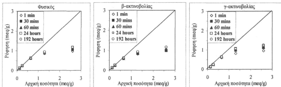
Σχήμα 4. Διάγραμμα ρόφησης \text{Cs}^+ σε σχέση με το χρόνο για φυσικό κλινοπτιλόλιθο, για τροποποιημένο κλινοπτιλόλιθο με ακτινοβολία ηλεκτρονίων και κλινοπτιλόλιθο τροποποιημένο με ακτινοβολία-γ. (άξονας x: αρχική ποσότητα γραμμοισοδυνάμων στο διάλυμα, άξονας y: γραμμοισοδύναμα τα οποία ροφήθηκαν, για όλες τις συγκεντρώσεις έγινε αναγωγή ανά γραμμάριο κλινοπτιλόλιθου)
