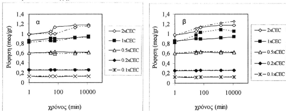
Σχήμα 2. Ρόφηση \text{Cs}^+ σε φυσικό κλινοπτιλόλιθο (συνεχής γραμμή) και α) σε κλινοπτιλόλιθο επεξεργασμένο με ακτινοβολία ηλεκτρονίων ( 10^{15} \text{ e/cm}^2 ) (διακεκομένη γραμμή) β) σε κλινοπτιλόλιθο επεξεργασμένο με ακτινοβολία-γ (70Mrad) (διακεκομένη γραμμή) (άξονας x: χρόνος αντίδρασης, άξονας y: γραμμοισοδύναμα τα οποία ροφήθηκαν, για όλες τις συγκεντρώσεις έγινε αναγωγή ανά γραμμάριο κλινοπτιλόλιθου)
