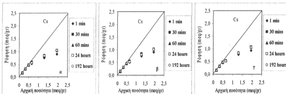
Σχήμα 8. Διαγράμματα ρόφησης \text{Cs}^+ σε σχέση με το χρόνο α) σε φυσικό κλινοπτιλολίθο, β) σε κλινοπτιλολίθο επεξεργασμένο με ακτινοβολία ηλεκτρονίων και γ) κλινοπτιλολίθο επεξεργασμένο με ακτινοβολία-γ. (άξονας x: αρχική ποσότητα γραμμοισοδυνάμων στο διάλυμα, άξονας y: γραμμοισοδύναμα τα οποία ροφήθηκαν, όλες οι συγκεντρώσεις είναι αναγόμενες ανά γραμμάριο κλινοπτιλολίθου)
