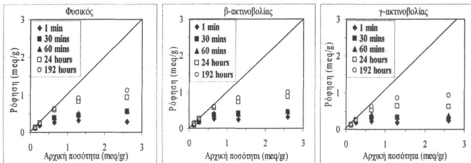
Σχήμα 5. Διαγράμματα ρόφησης \text{Sr}^{2+} σε σχέση με το χρόνο για φυσικό κλινοπτιλόλιθο, για κλινοπτιλόλιθο επεξεργασμένο με ακτινοβολία ηλεκτρονίων και κλινοπτιλόλιθο επεξεργασμένο με ακτινοβολία-γ. (άξονας x: αρχική ποσότητα γραμμοισοδυνάμων στο διάλυμα, άξονας y: γραμμοισοδύναμα τα οποία ροφήθηκαν, για όλες τις συγκεντρώσεις έγινε αναγωγή ανά γραμμάριο κλινοπτιλόλιθου)
