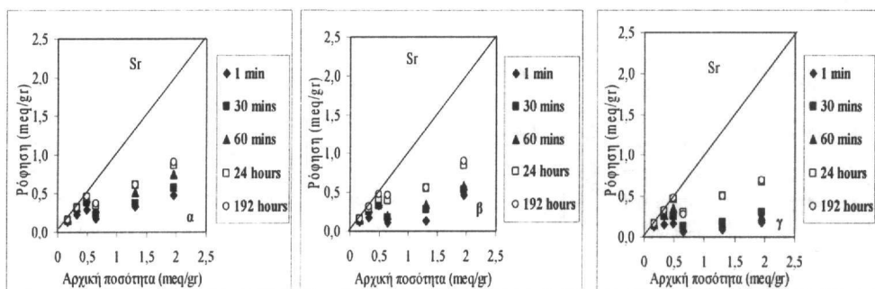
Σχήμα 9. Διαγράμματα ρόφησης \text{Sr}^{2+} σε σχέση με το χρόνο α) σε φυσικό κλινοπτιλολίθο, β) σε κλινοπτιλολίθο επεξεργασμένο με ακτινοβολία ηλεκτρονίων και γ) σε κλινοπτιλολίθο επεξεργασμένο με ακτινοβολία-γ. (άξονας x: αρχική ποσότητα γραμμοισοδυνάμων στο διάλυμα, άξονας y: γραμμοισοδύναμα τα οποία ροφήθηκαν, όλες οι συγκεντρώσεις είναι αναγόμενες ανά γραμμάριο κλινοπτιλολίθου)
