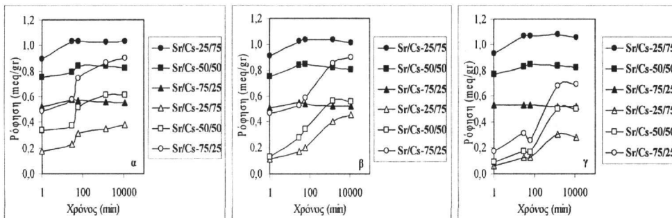
Σχήμα 6. Ρόφηση Cs + (μαύρα σύμβολα) και Sr 2+ (κενά σύμβολα) α) σε φυσικό κλινοπυλλοίθιο β) σε κλινοπυλλοίθιο επεξεργασμένο με ακτινοβολία ηλεκτρονίων (10 14 e/cm 2 ) γ) σε κλινοπυλλοίθιο επεξεργασμένο με ακτινοβολία-γ (70Mrad). Τα ίδια σχήματα αναφέρονται σε διαλύματα αντίστοιχων αναλογιών για παράδειγμα ο μαύρος κύκλος αναφέρεται σε διάλυμα αναλογίας Cs + /Sr 2+ =75/25 και ο κενός κύκλος σε διαλύματα Sr 2+ /Cs + =75/25. Συγκέντρωση διαλύματος 2xCEC.
