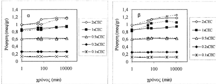
Σχήμα 2. Ρόφηση Cs + σε φυσικό κλινοπτιλόλιθο (συνεχής γραμμή) και α) σε κλινοπτιλόλιθο επεξεργασμένο με ακτινοβολία ηλεκτρονίων (10 15 e/cm 2 ) (διακεκομμένη γραμμή) β) σε κλινοπτιλόλιθο επεξεργασμένο με ακτινοβολία-γ (70Mrad) (διακεκομμένη γραμμή) (άξονας x: χρόνος αντίδρασης, άξονας ψ: γραμμοισοδύναμα τα οποία ροφήθηκαν, για όλες τις συγκεντρώσεις έγινε αναγωγή ανά γραμμάριο κλινοπτιλόλιθου)
