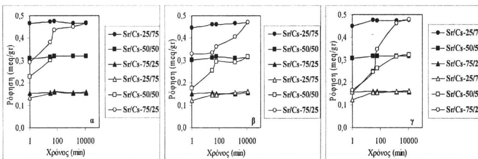
Σχήμα 7. Ρόφηση Cs + (μαύρα σύμβολα) και Sr 2+ (κενά σύμβολα) α) σε φυσικό κλινοπυλλοίθιο β) σε κλινοπυλλοίθιο επεξεργασμένο με ακτινοβολία ηλεκτρονίων (10 14 e/cm 2 ) γ) σε κλινοπυλλοίθιο επεξεργασμένο με ακτινοβολία-γ (70Mrad). Τα ίδια σχήματα αναφέρονται σε διαλύματα αντίστοιχων αναλογιών για παράδειγμα ο μαύρος κύκλος αναφέρεται σε διάλυμα αναλογίας Cs + /Sr 2+ =75/25 και ο κενός κύκλος σε διαλύματα Sr 2+ /Cs + =75/25. Συγκέντρωση διαλύματος 0,5xCEC.
