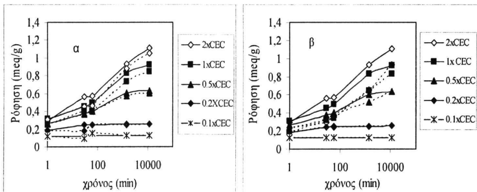
Σχήμα 3. Ρόφηση Sr 2+ σε φυσικό κλινοπτιλόλιθο (συνεχής γραμμή) και α) σε κλινοπτιλόλιθο επεξεργασμένο με ακτινοβολία ηλεκτρονίων (10 15 e/cm 2 ) (διακεκομμένη γραμμή) β) σε κλινοπτιλόλιθο επεξεργασμένο με ακτινοβολία γ (70Mrad) (διακεκομμένη γραμμή) (άξονας x: χρόνος αντίδρασης, άξονας ψ: γραμμοισοδύναμα τα οποία ροφήθηκαν, για όλες τις συγκεντρώσεις έγινε αναγωγή ανά γραμμάριο κλινοπτιλόλιθου)
