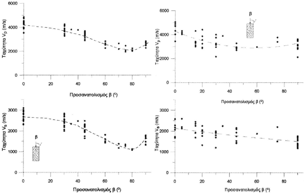
Σχήμα 1. Διάγραμμα ταχύτητας διάδοσης επιμήκων ( V_p ) και εγκάρσιων κυμάτων ( V_s ) του γνευσιού (αριστερά) και του σχιστόλιθου (δεξιά) σε σχέση με τη γωνία \beta που σχηματίζει ο άξονας φόρτισης με τα επίπεδα σχιστότητας
