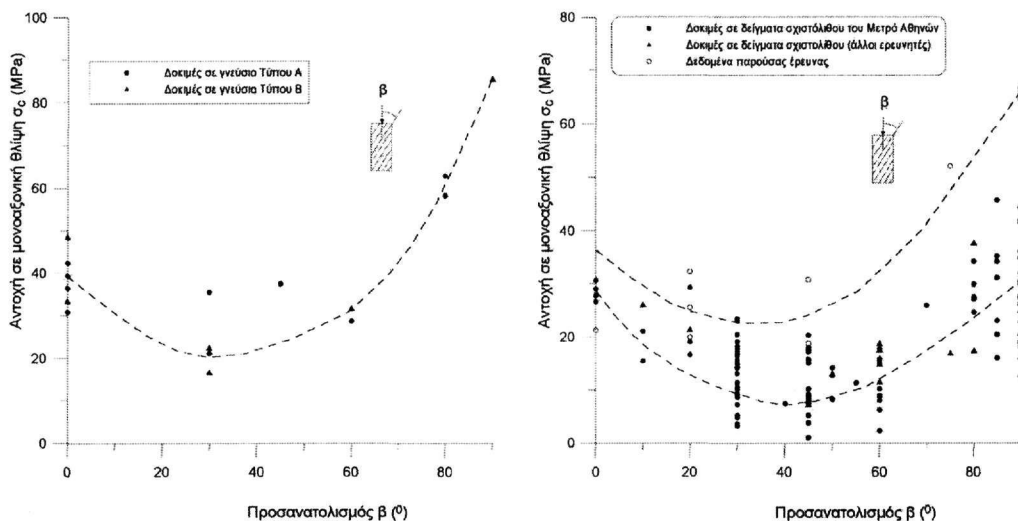
Σχήμα 2. Διάγραμμα αντοχής σε μονοαξονική θλίψη ( \sigma_c ) του γνευσίου (αριστερά) και του σχιστολίθου (δεξιά) σε σχέση με τη γωνία \beta που σχηματίζει ο άξονας φόρτισης με τα επίπεδα σχιστότητας
