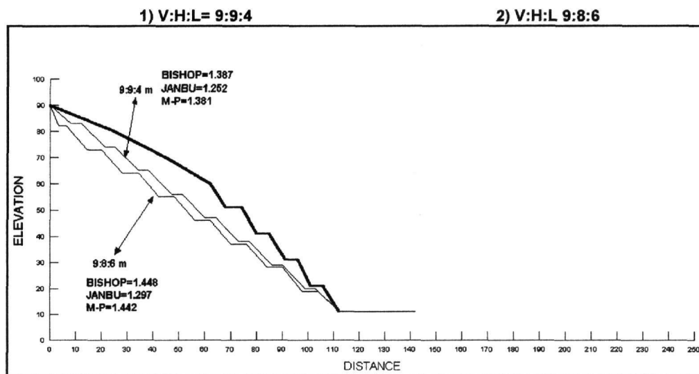
Σχ. 18. Συγκριτική παρουσίαση των 2 ευνοϊκότερων μορφολογιών με βάση την γεωμετρία των αναβαθμιδών.
