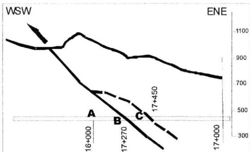
Σχ. 7 Σχηματική ανάπτυξη της επώθησης
