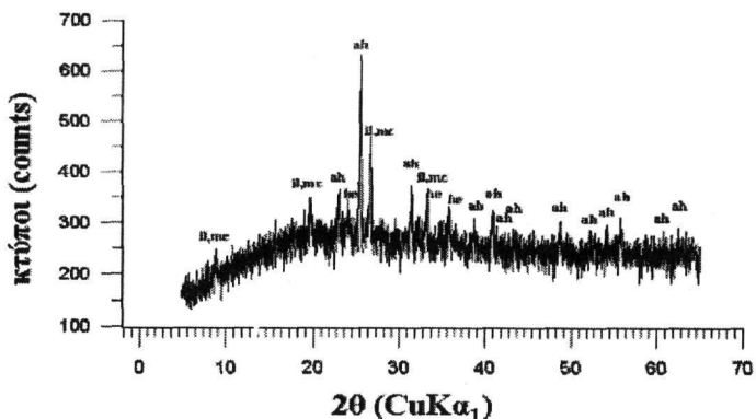
Σχήμα 3. Ακτινογράφημα της τέφρας (750 o C) του δείγματος ΚΠ-13/5 (il,mc: ιλλίτης, μαρμαρυγίες, ah: ανυδρίτης, he: αιματίτης).
