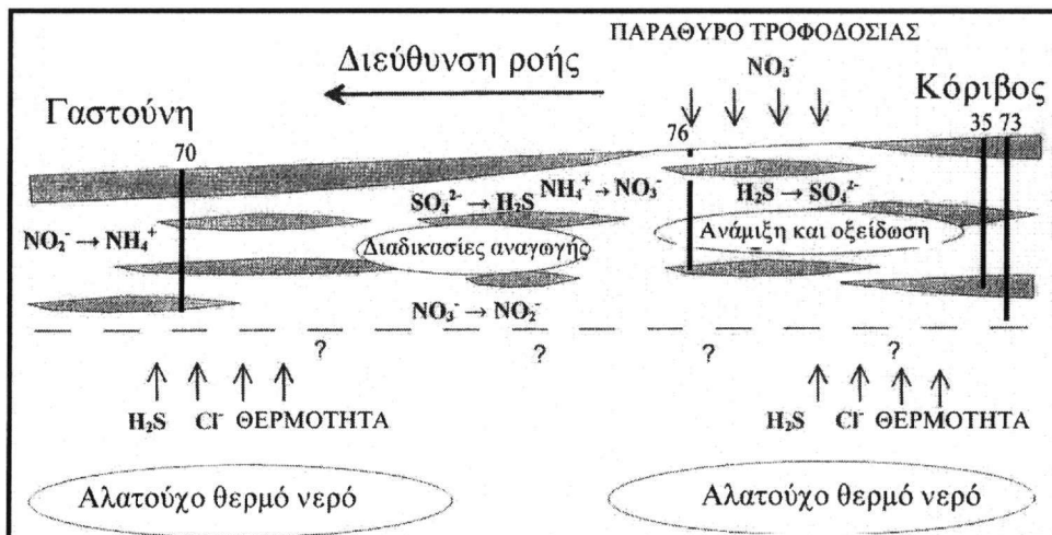
Σχήμα 6: Σχηματική υδρογεωλογική - υδροχημική τομή κατά μήκος της γραμμής ροής Α (βλ. Σχ. 2α)
