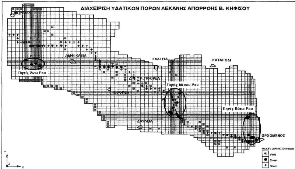
Σχήμα 2. Κάναβος μαθηματικού ομοιώματος και οριακές συνθήκες. Με ελλείψεις σημειώνονται οι ζώνες ανάπτυξης των καρστικών πηγών.
