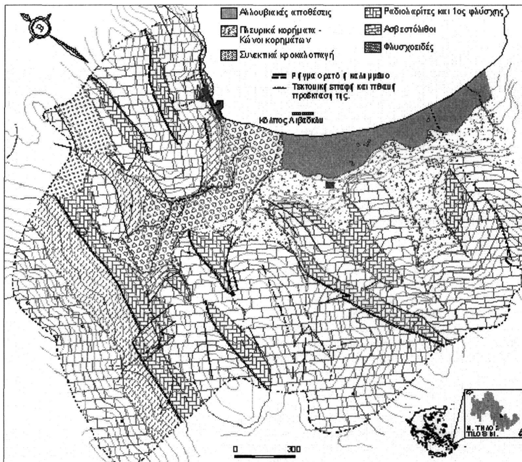
Σχήμα 1. Γεωλογικός χάρτης ευρύτερης περιοχής Λιβαδιών Τήλου
