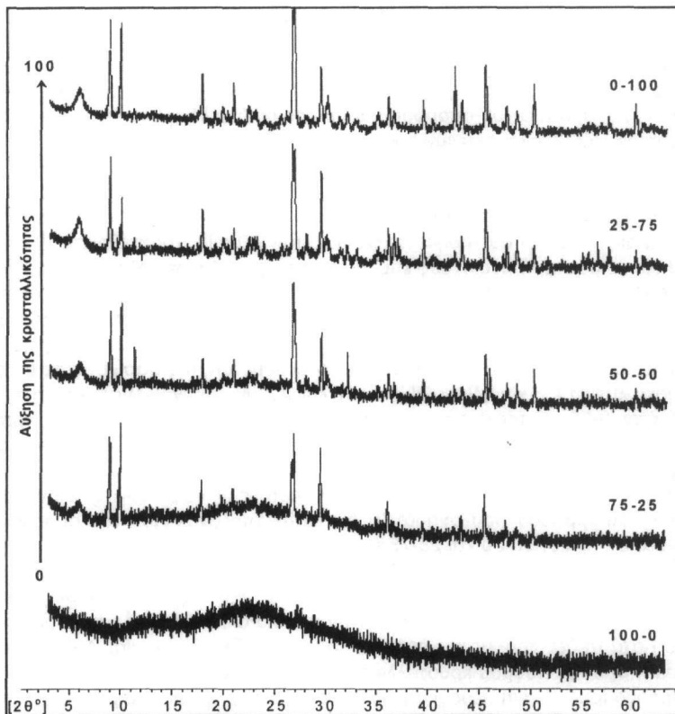
Σχήμα 1. Περιθλασιογράμματα των πρότυπων μιγμάτων.
