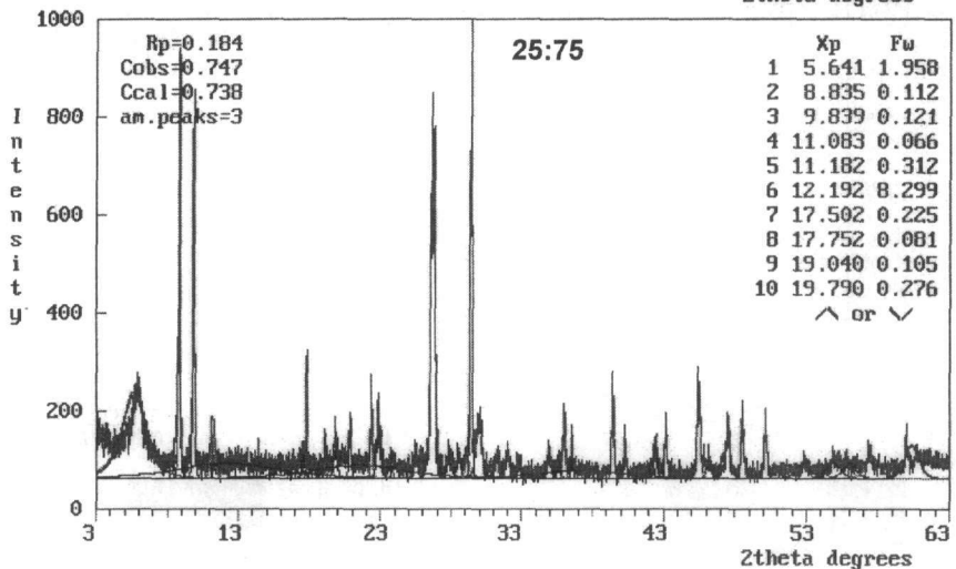
Σχήμα 3. Υπολογισμός της κρυσταλλικότητας.
