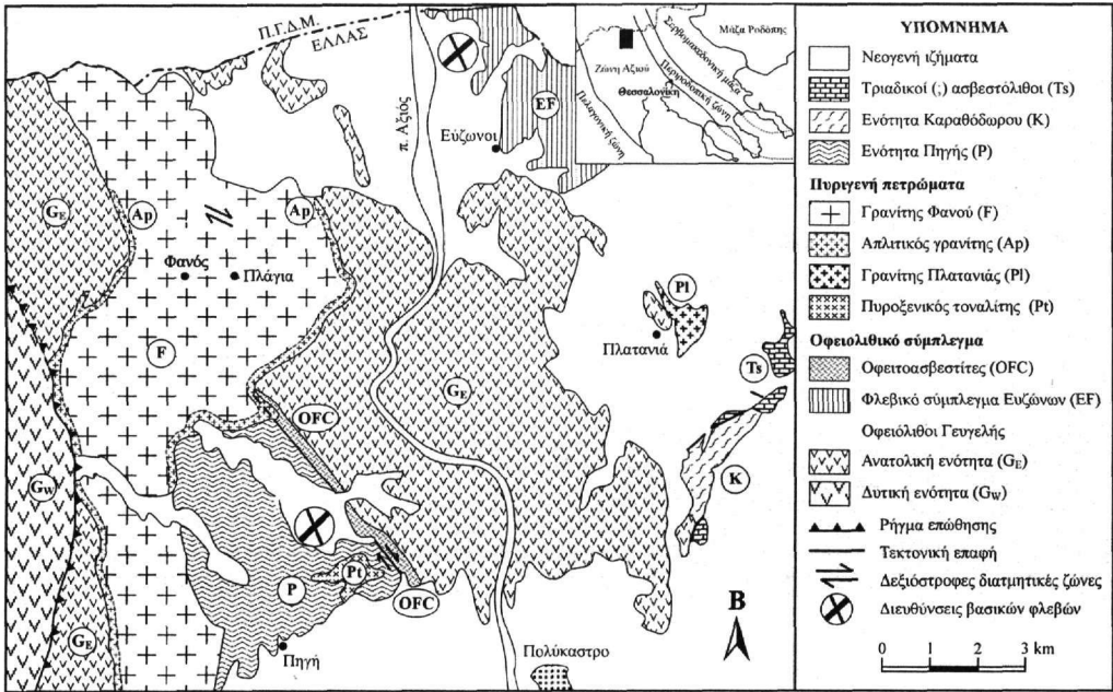
Σχήμα 1. Γεωλογικός χάρτης (βασισμένος σε Mercier 1968, Bebien 1982, ΙΓΜΕ 1982, 1993 και σε δικά μας δεδομένα) του βορειότερου τμήματος της ζώνης Stip-Αζίου στον ελληνικό χώρο. Στο χάρτη σημειώνονται οι ενότητες Πηγής (P) και Καραθόδωρου (K).
