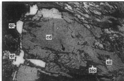
Σχήμα 4 (αριστερά). Κορώνες κορδιερίτη (cd) γύρω από γρανάτη (gt) στα μεσοσώματα των μεταίζημάτων. Η επίπεδη υφή που ορίζεται από ινώδη σιλλιμανίτη (sil) και βιοτίτη (bio) κάμπτεται γύρω από τον κρύσταλλο του γρανάτη. Παράλληλα Nicols. Η μεγάλη πλευρά της φωτογραφίας αντιστοιχεί σε 2.30 mm.
