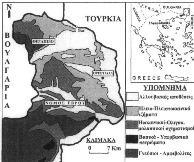
Σχήμα 1. Απλοποιημένος γεωλογικός χάρτης της περιοχής του Νόμου Έβρου, (Α. Kassoli – Foyrparaki et al. 1995, τροποποιημένος από Χ. Κανελλόπουλο 2004).
