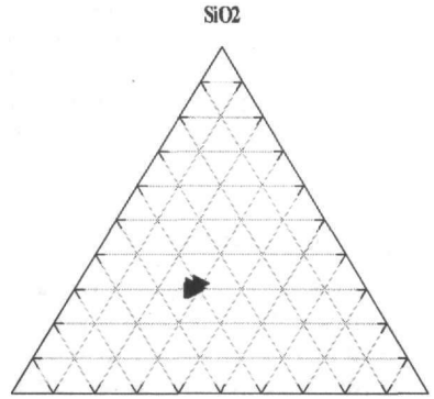
Σχήμα 4. Προβολή της σύστασης του τιτανίτη στο διάγραμμα SiO_2 - TiO_2 - CaO .
