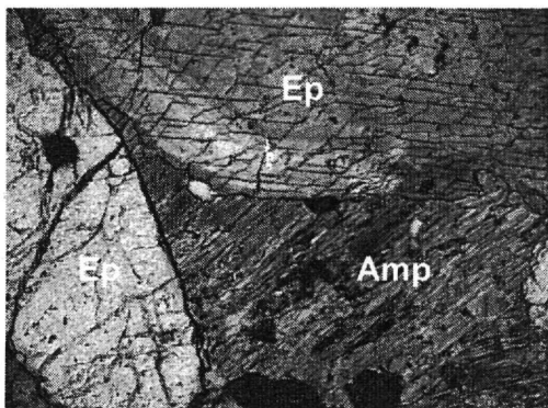
Σχήμα 2. Κροστίλβη (εξαλλοίωση προς βιοτίτη). x80 κάθετα nicols, (Amp = αμφίβολος, Ep = Επίδοτο)
