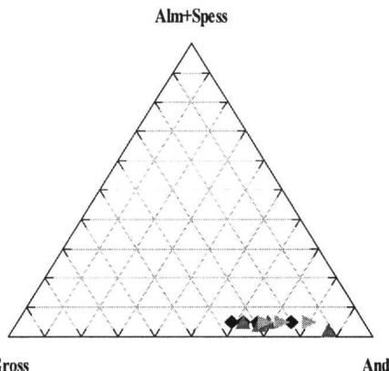
Σχήμα 11. Προβολή των γρανατών του skarn στο διάγραμμα Alm+Spess – Gross – And
