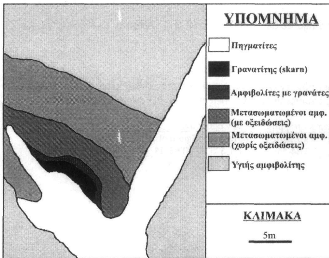
Σχήμα 8. Γεωλογικό σκαρίφημα του skarn στο Θεραπειό.
