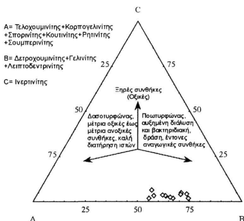
Σχήμα 4. Προβολή των πιμών Α, Β, C των δειγμάτων του λιγνίτη από τον Δυτικό τομέα, στο διάγραμμα Μυκο- radhyay (1989).
