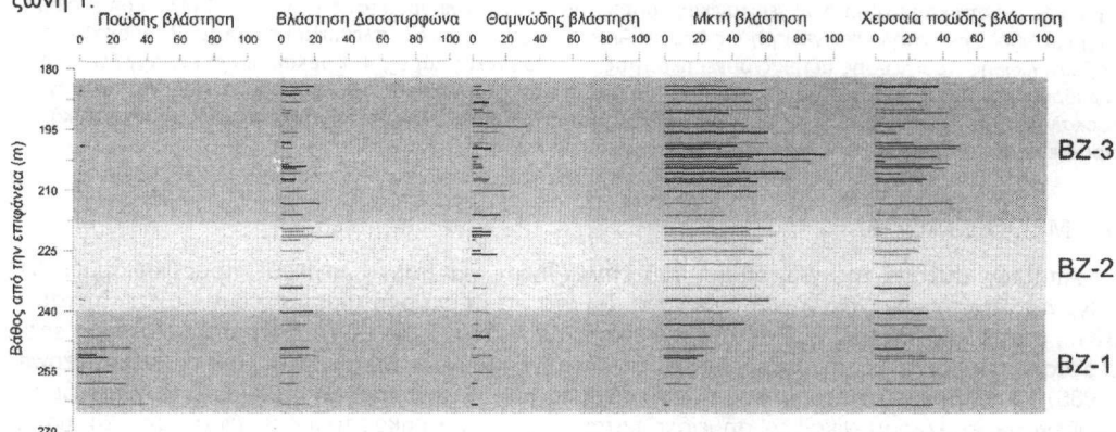
Σχήμα 2. Συνοπτικό παλυνολογικό διάγραμμα της γεώτρησης #53. Πωώδης ελόβια Βλάστηση: Cyperaceae , Typhaceae , Sparganiaceae , Carex , Nymphaeaceae , Liliaceae , Βλάστηση Δασοτυρφώνα: Taxodium , Nyssa , Θαμνώδης Βλάστηση: Myricaceae , Salix , Alnus , Betula , Μικτή Βλάστηση: Pinus , Sciadopitys , Symplocos , Palmae , Carya , Pterocarya , Vitis , cf. Quercus , Quercus coccifera -type, Ilex , Ulmus / Zelkova , Fagus , Fraxinus , Buxus , Quercus pubescens , Acer , Carpinus , Oleaceae , Sapotaceae , Engelhardtia , Χερσαία πωώδης Βλάστηση: Graminae , Compositae , Chenopodiaceae / Amaranthaceae , Cruciferae , Umbelliferae , Ephedra , Artemisia , Rubiaceae , Parthenocissus , Myriophyllum , Osmundaceae , Polypodiaceae .
