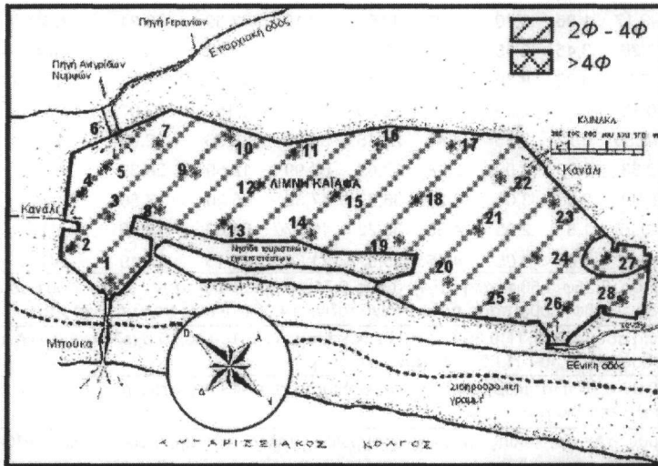
Σχήμα 6. Η χωρική κατανομή του αποκλειστικού γραφικού βαθμού ταξινόμησης (σι).
