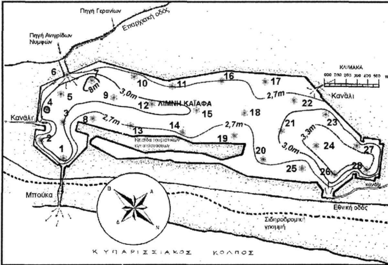
Σχήμα 2. Σχηματικό σκαρίφημα βαθυμετρικού χάρτη Λθ Καϊάφα, με τις θέσεις επιφανειακής δειγματοληψίας.
