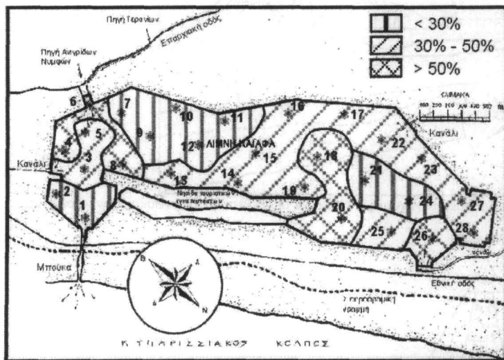
Σχήμα 4. Η ποσοτική χωρική κατανομή του κλάσματος της άμμου στη λιμνοθάλασσα του Καϊάφα.
