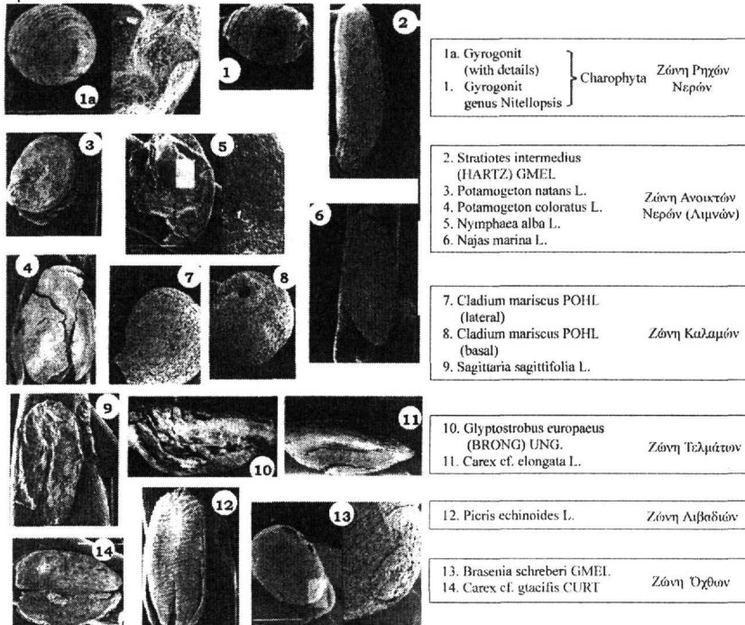
Σχήμα 1. Σπέρματα και καρποί από λιγνιτικά κοιτάσματα του ελλαδικού χώρου.
