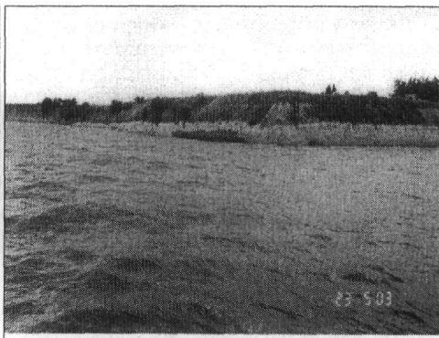
Σχήμα 10. Υψηλές ακτές Ν. Κεσσάνης
