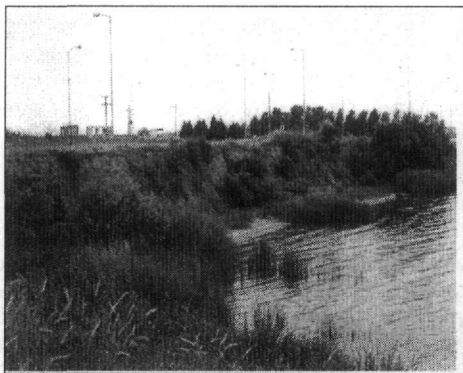
Σχήμα 6. Υψηλές ακτές της περιοχής Γλυκονερίου
