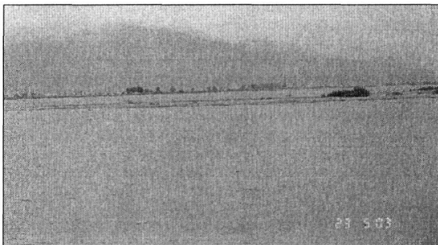
Σχήμα 5. Σχηματισμός αμμώδη βραχίονα στις εκβολές Κομφάτου ΒΔ τμήμα της λίμνης Βιστωνίδας
