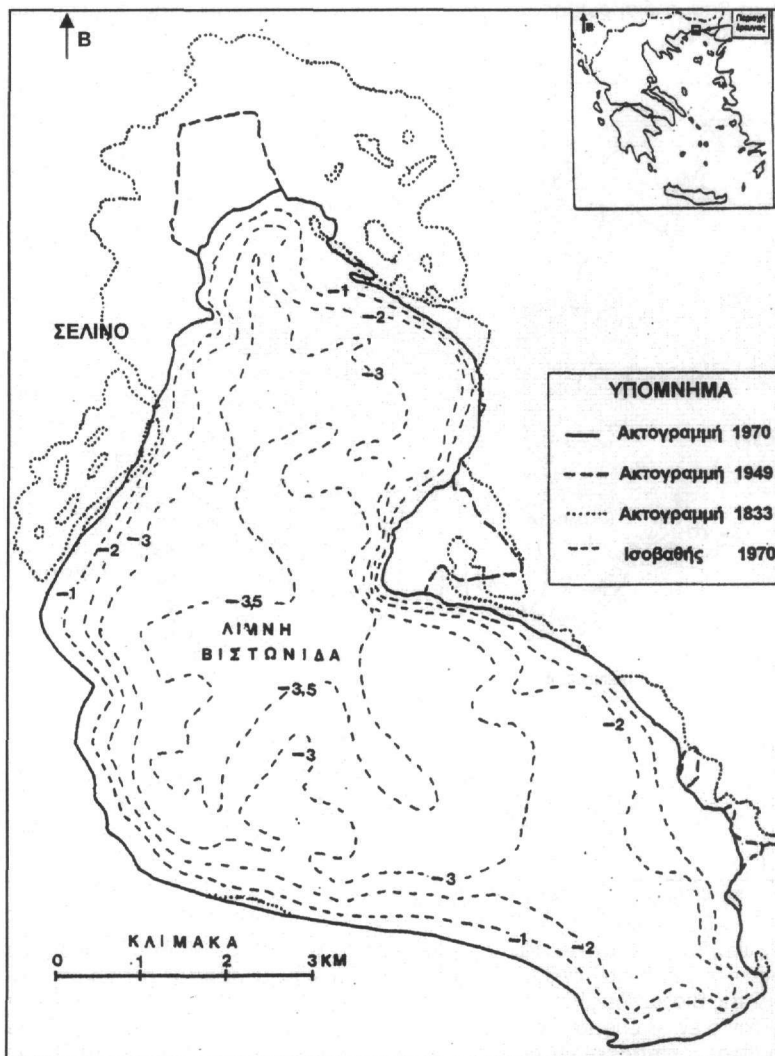
Σχήμα 4. Χάρτης μεταβολής της ακτογραμμής της λίμνης Βιστωνίδα για τα έτη 1833, 1949 και 1970. Ισοβαθείς 1970.
