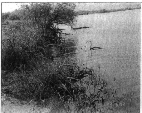
Σχήμα 11. Διαβρωσιγενείς ακτές περιοχής Σέλιου
