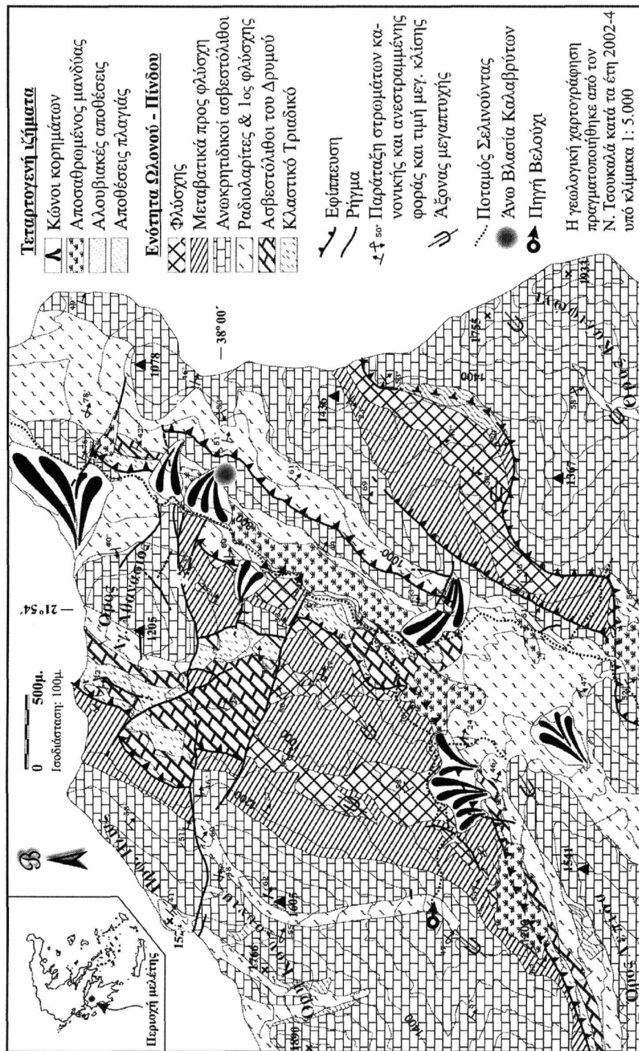
Σχήμα 1. Γεωλογικός χάρτης του βορείου τμήματος της υδρολογικής λεκάνης του άνω ρου του ποταμού Σελινούντα (Ν. Αχΐας)
