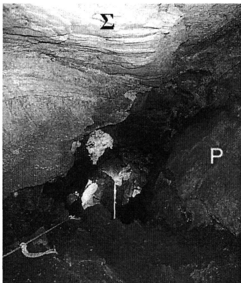
Σχήμα 6. Το κεκλιμένο σπήλαιο ανατολικά από τη θέση Γεράκι. Διακρίνεται η κατοπτρική επιφάνεια του ρήγματος (Ρ) με στοιχεία 71^{\circ}038' , αλλά και η στρώση (Σ) των τριαδικών ασβεστολίθων «του Δρυμού».
