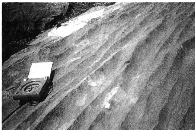
Σχήμα 3. Γλυφές οι οποίες έχουν δημιουργηθεί παράλληλα με την επιφάνεια στρώσης των μεταβατικών ιζημάτων προς τον φλύσχη.
