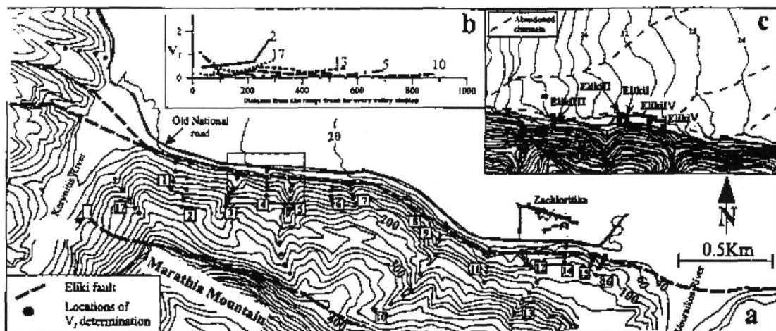
Σχ.3 (α) Μορφοτεκτονικός χάρτης της περιοχής, που δείχνει τη ρηξιγενή ζώνη της Ελίκης και το σύστημα αποστράγγισης κατά μήκος του πρηνούς του ρήγματος. Τα έντονα νούμερα δείχνουν τις ισοψείες με ισοδιάσταση 100m και τα αριθμημένα πλαίσια απεικονίζουν τα ρέματα που αποστραγγίζουν το πρηνές του ρήγματος. (β) Διάγραμμα που δείχνει δεδομένα V_f στα πέντε μεγαλύτερα ρέματα αποστράγγισης του πρηνούς του ρήγματος. Το νούμερο στο διάγραμμα αντιστοιχεί στα αριθμημένα ρέματα του μορφοτεκτονικού χάρτη. (γ) Λεπτομερής τοπογραφικός χάρτης με ισοδιάσταση τεσσάρων μέτρων που δείχνει την τοποθεσία των τομών (μαύρα ορθογώνια) και τους αποξηραμένους παραποτάμους του Κερυνίτη ως διακεκομμένες γκριζές γραμμές. Fig. 3 (a) Morphotectonic map of the study area, showing the Heliki fault zone and drainage pattern across the fault scarp. The rectangle shows the area of the detailed topographic map. (b) Diagram showing V_f data in the five longer streams draining the fault scarp. Number in the diagram corresponds to the numbered streams on the morphotectonic map. (c) Detailed topographic map, contouring at 4 meters interval, showing the location of trenches as solid parallelograms and abandoned branches of the Kerynites river as dashed grey lines.
