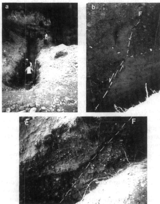
Σχ.4 Φωτογραφία (a): Η εκσκαφή (τομή) IV (Ιούλιος 2000) σε γενική άποψη. (b): Λεπτομέρεια του ρήγματος με άλμα που επηρεάζει τις άμμους και τα κροκαλοπαγή (ποτάμιες αποθέσεις) και στο πάνω αριστερό άκρο διακρίνεται μία «κολλουβιακή σφήνα». (c) : Λεπτομέρεια από την τομή V όπου φαίνεται η μετατόπιση των παλαιοκροκαλοπαγών του Κερυνίτη. Κάναβος 1x1 m. (F=Ρήγμα)
