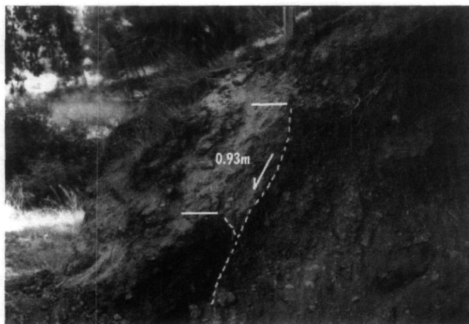
Σχ.7: Η κατακόρυφη μετατόπιση (άλμα) 0.93m μεταξύ του κροκαλοπαγούς της βάσης (Brick orange fluvial deposits, Koukouvelas et al 2001), παλαιοεδάφους (palaeosoil) ηλικίας 750 χρόνων ( C_{14} ) και νεότερων πλεονεκτών κορημάτων (colluvium+soil), όπως αποκαλύφθηκε στην εκσκαφή I.
