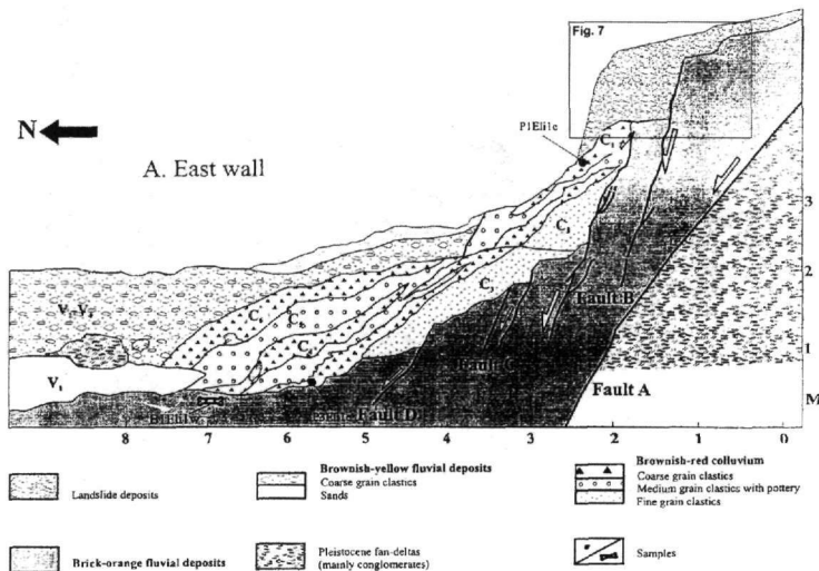
Σχ.5: Η παλαιοσεισμολογική τομή I σε σκίτσο μετά από αποτύπωση σε κλίμακα 1:20. Fault A: Περιθωριακό κύριο ρήγμα Ελίκης. Fault B: Το πρώτο ρήγμα-διάρρηξη του σεισμού του 1861. Fault C-D: Παλαιότερης δραστηριοποίησης. (N= βορράς)
