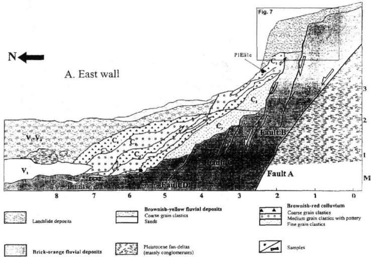
Σχ.5: Η παλαιοσεισμολογική τομή I σε σκίτσο μετά από αποτύπωση σε κλίμακα 1:20. Fault A: Περιθωριακό κύριο ρήγμα Ελέκης. Fault B: Το πρώτο ρήγμα-διάρρηξη του σεισμού του 1861. Fault C-D: Παλαιότερης δραστηριοποίησης. (N= βορράς)
