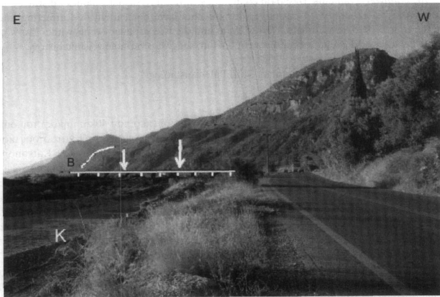
Σχ.2 Φωτογραφία του Ανατολικού τμήματος του ρήγματος της Ελίκης, μεταξύ των ποταμών Κερυνίτη (Κ) και Βουραικού (Β). Με βέλη δείχνονται οι θέσεις των παλαιοσεισμικών εκσκαφών. Fig.2 Photograph that shows the eastern part of the Heliki fault, between the rivers Kerynites (K) and Vouraikos (B). The arrows show the palaeoseismological trenches.
