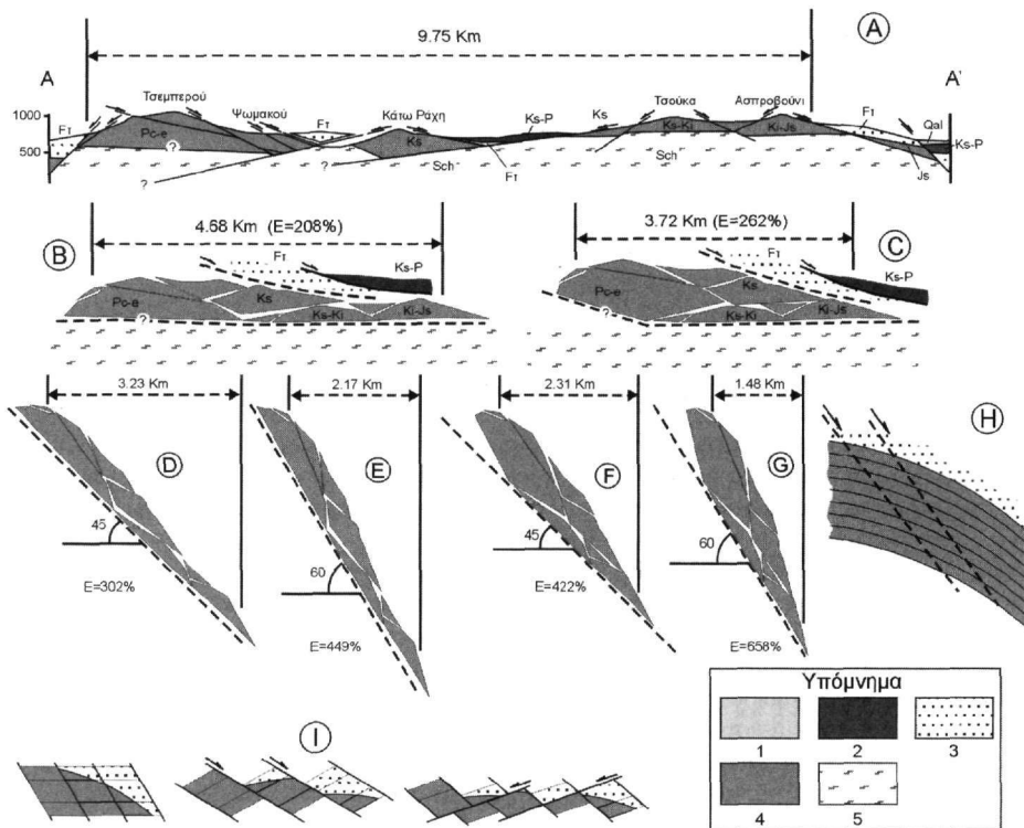
Εικ. 3: (A) Η τομή AA' της εικ. 1. (B, C) Δύο περιπτώσεις ανακατασκευής της τομής ανάλογα αν τα ΒΑ διεύθυνσης ρήγματα της Τσεμπερούς αποτελούν ή όχι τη συνέχεια των ίδιας διεύθυνσης ρηγμάτων της Τσοούκα και Ασπροβουνίου. (D, E, F, G) Η γεωμετρία της ανθρακικής ακολουθίας της Τρίπολης πριν αυτή διαρρηχθεί σε περίπτωση που το ρήγμα ΒΛΚ ήταν ένα μεγάλης κλίσης κανονικό ρήγμα. Σε μία τέτοια περίπτωση οι ανθρακικές μάζες της τομής AA' αποτελούσαν τμήμα μίας μεγάλης κλίμακας αντικλινικής δομής (H). (I) Μοντέλο εφελκυστικής παραμόρφωσης της ανώτερης πλάκας. 1. Αλλούβια, 2. Ανωκρητιδικό ασβεστόλιθο της ενότητας Πίνδου (Ks-P), 3. Φλύσχης Τρίπολης (Fr), 4. Ασβεστόλιθοι Τρίπολης, 5. Φυλλίτες-Χαλαζίτες (Sch). Fig. 3: (A) AA' cross section of fig. 1. (B, C) Two different cases depending on the continuity or not of the NW-oriented faults of Tsemberou to Tsouka or Asprovouni faults. The geometry of Tripolis Unit's limestones just before been faulted in the case that VLK fault was a high-angle normal fault. In such a case the limestones depicted in AA' cross section belonged to a macroscale anticline (H). (I) Deformation model of the upper plate. 1. Alluvial, 2. Limestones of U. Cretaceous age of Pindos Unit (Ks-P), 3. Flysch of Tripolitza Unit (Fr), 4. Limestones of Tripolitza Unit, 5. Phyllites-Quartzites (Sch).
