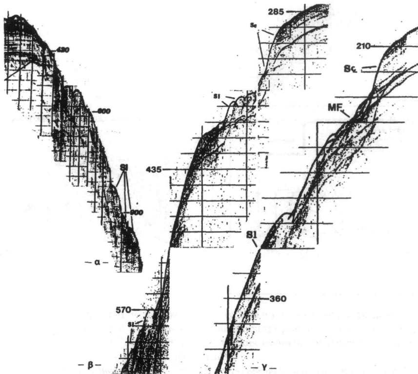
Εικ. 3: Τομογραφίες τύπου Sparker (α) και 3.5kHz (β) στην πλαγιά των ΝΝΑ-ικών Παξών και τύπου 3.5kHz στην πλαγιά της Κέρκυρας (γ) στις οποίες φαίνονται ολισθήσεις ιζηματογενών τεμαχών (SI), επιφάνειες αποκόλλησης (Sc) και επικαλυπτόμενες αποθέσεις βαρυτικών ροών (MF).
