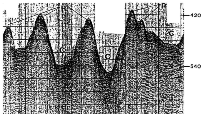
Εικ. 2: Τομογραφία τύπου Sparker στην οποία φαίνονται οι εναλλαγές υποθαλάσσιων χαραδρώσεων (C) και ράχων (R) στην πλαγιά των ΝΝΑ-ικών Παξών.
